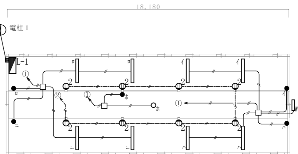
1号廠舎電灯設備改修平面図 1:150
