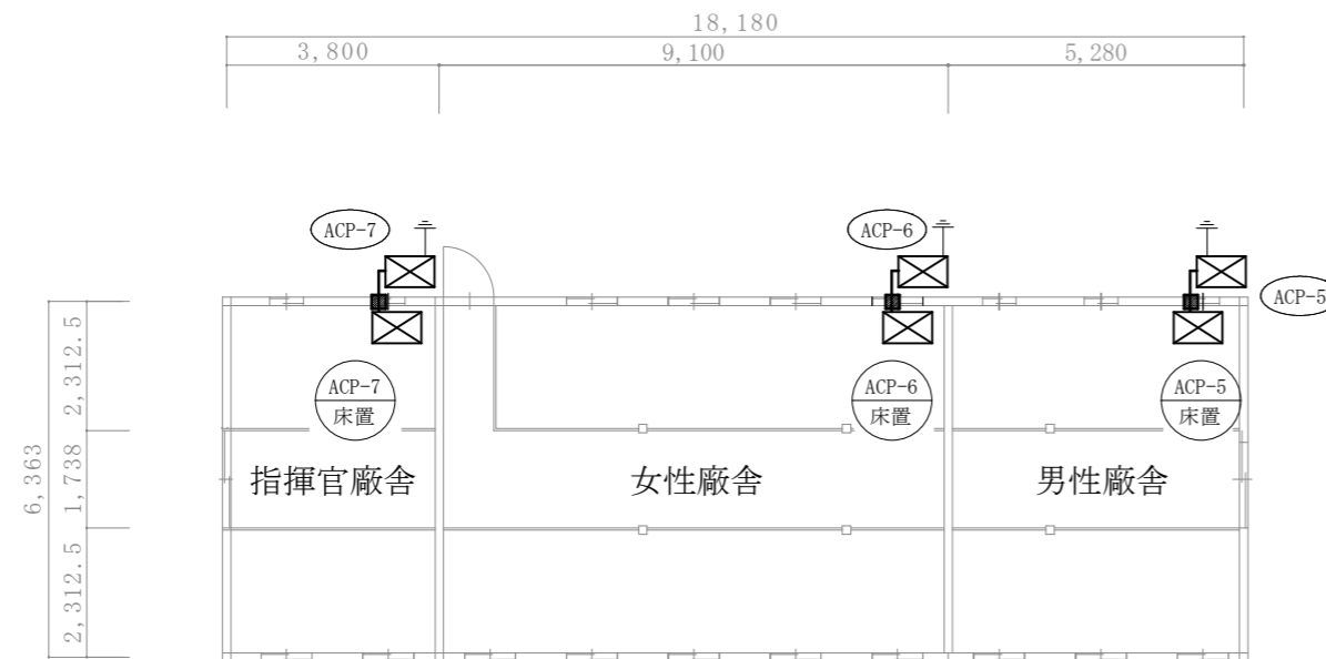
3号廠舎空調設備改修平面図 1:150
