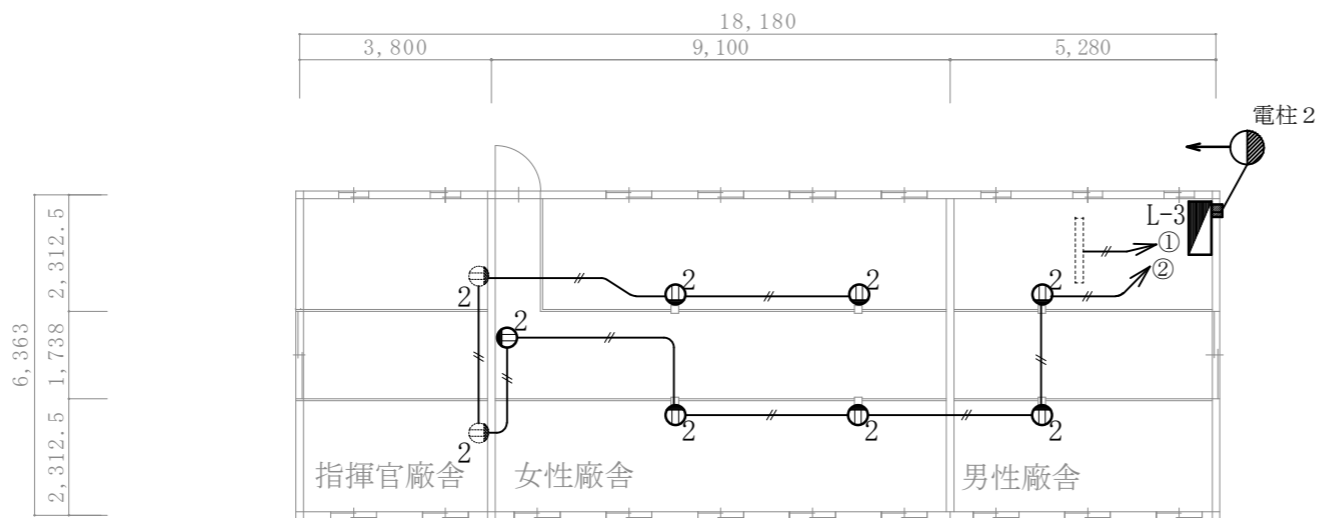
3号廠舎電気設備既設平面図 1:150
