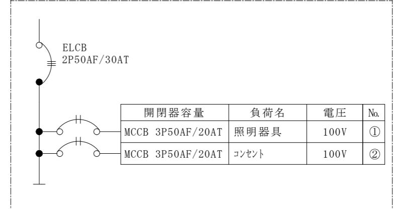
新設電灯分電盤 (L-2)
