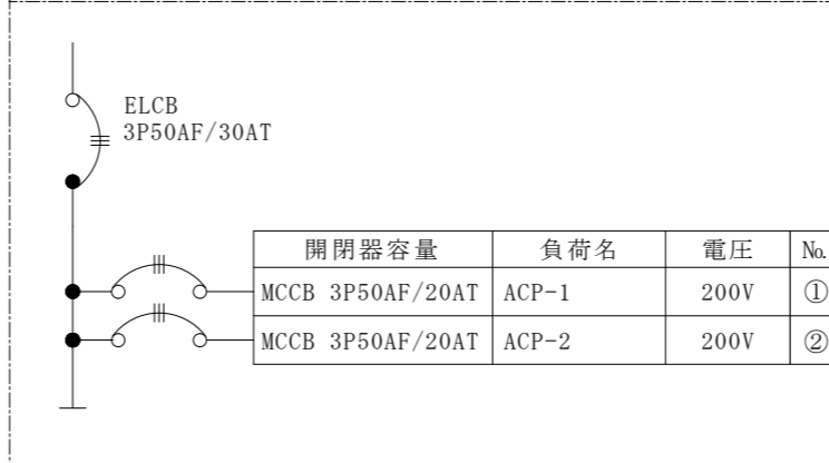
新設動力分電盤 (P-2)
