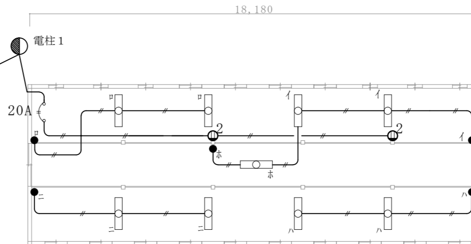
1号廠舎電灯設備既設平面図 1:150
