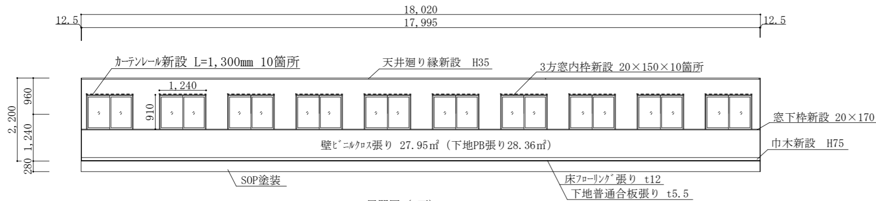
展開図 (C面) 1:100
