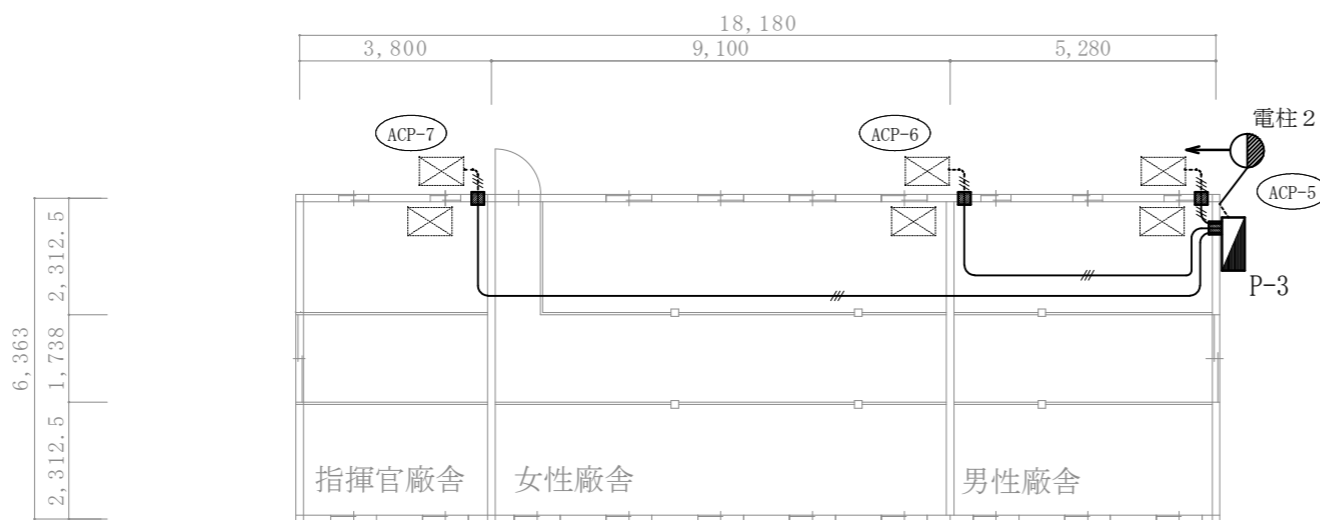
3号廠舎動力設備改修平面図 1:150
