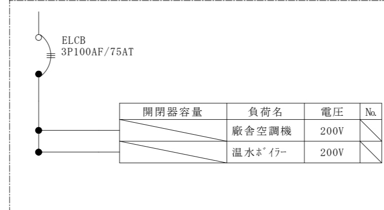
新設動力分電盤 (P-1)
