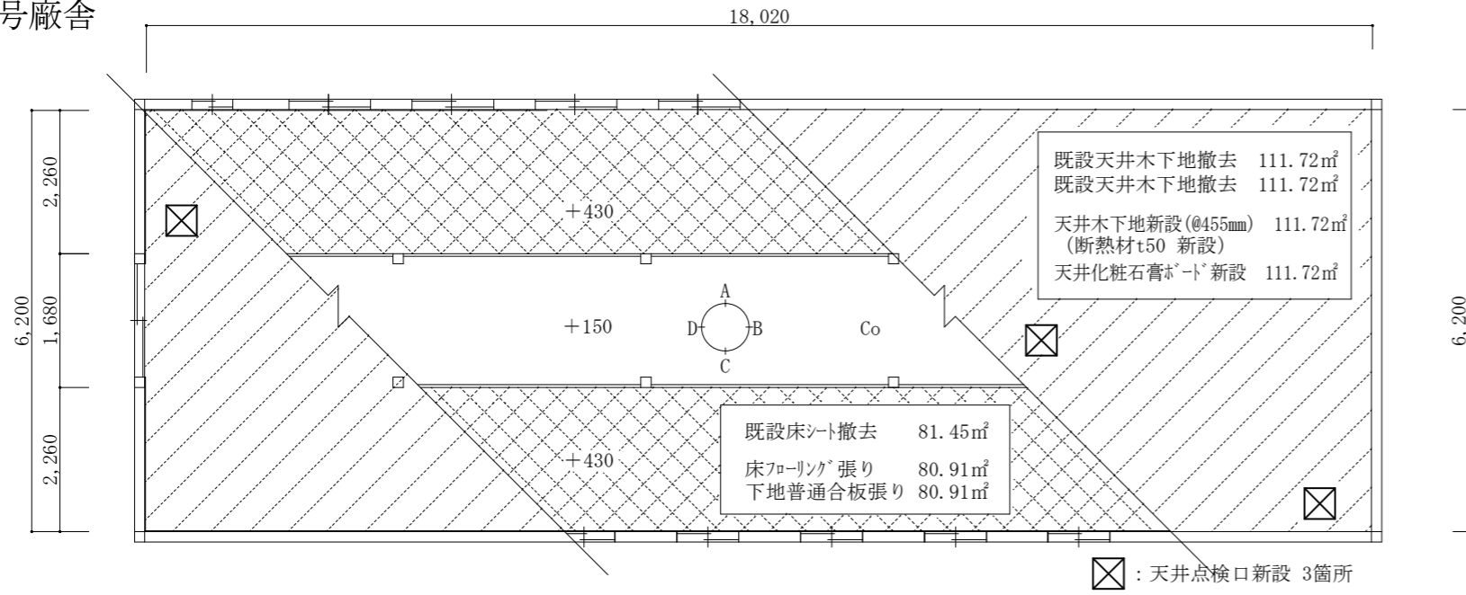
1号廠舎改修平面図・天井伏図 1:100
