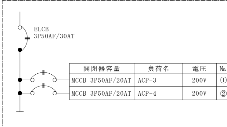
新設動力分電盤 (P-3)
