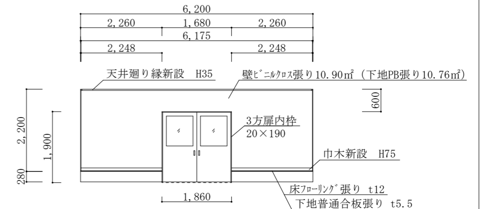
展開図 (D面) 1:100
