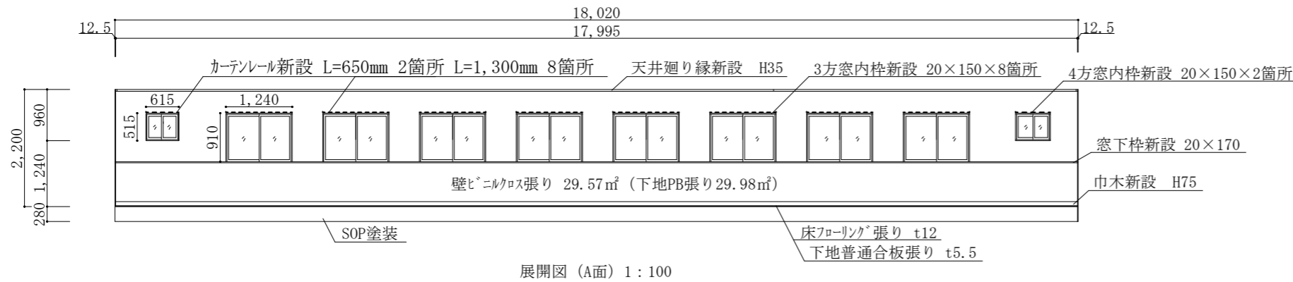
展開図 (A面) 1:100
