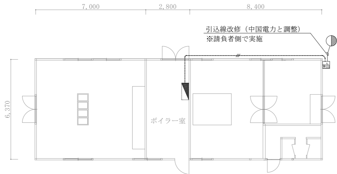
浴場動力設備既設平面図 1 : 150
