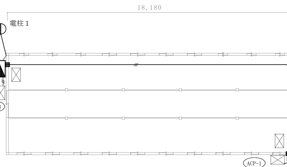
1号廠舎動力設備改修平面図 1:150
