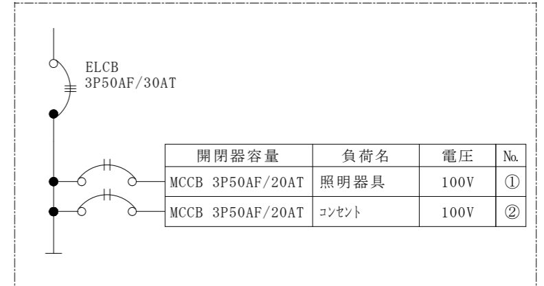
新設電灯分電盤 (L-3)
