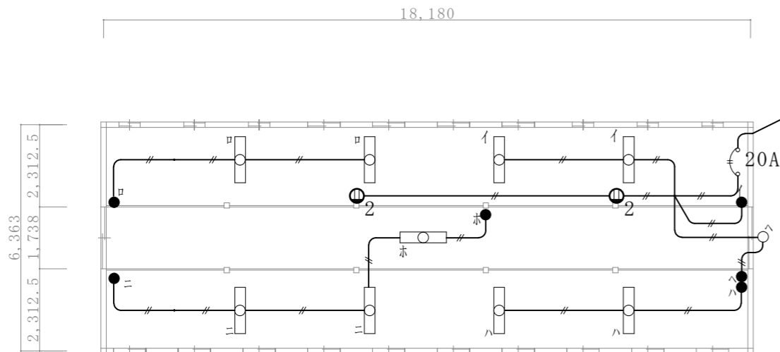
2号廠舎電灯設備既設平面図 1:150
