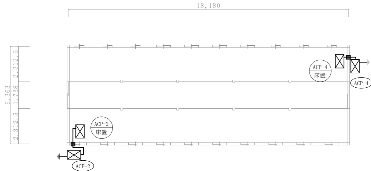
2号廠舎空調設備改修平面図 1:150
