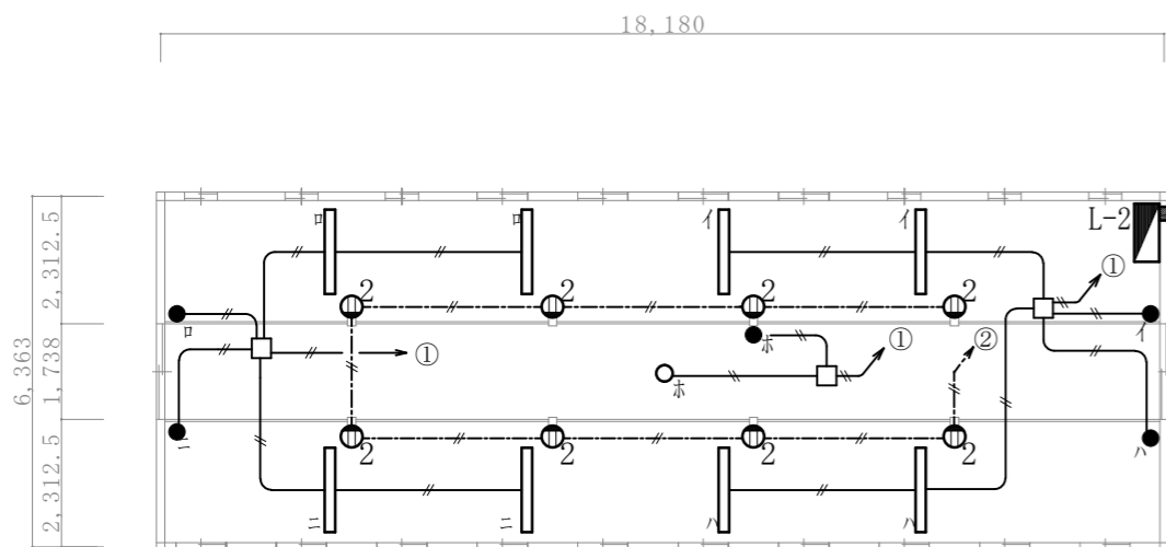
2号廠舎電灯設備改修平面図 1:150
