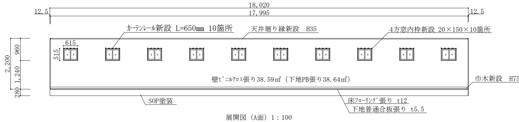
展開図 (A面) 1:100
