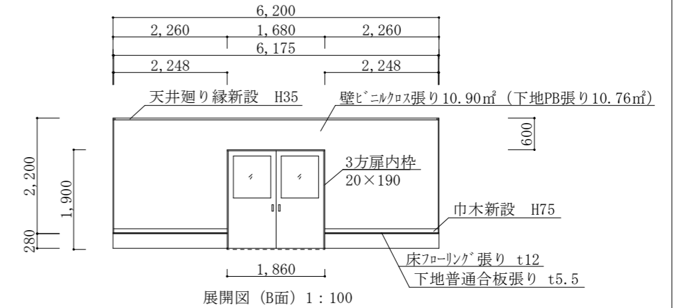
展開図 (B面) 1:100
