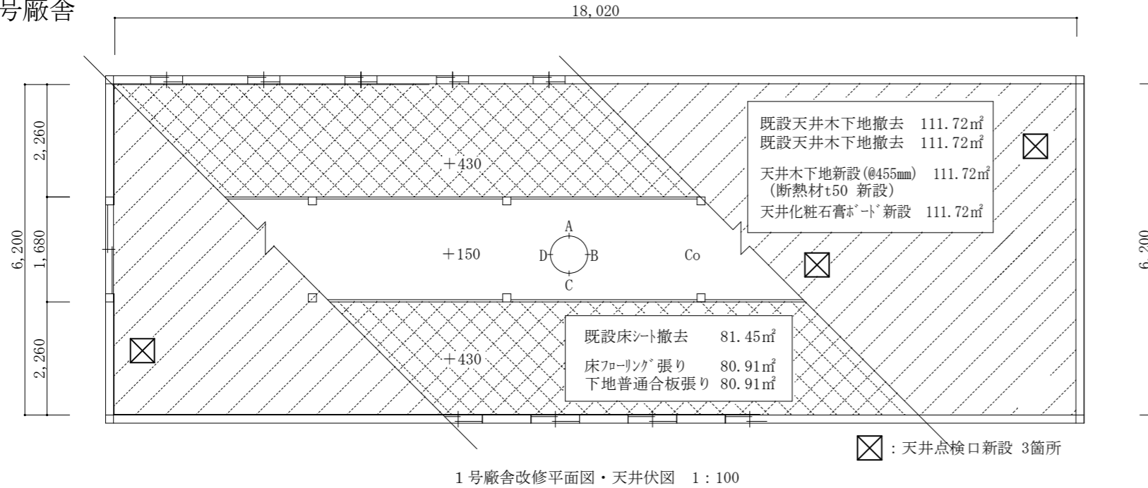
1号廠舎改修平面図・天井伏図 1:100
