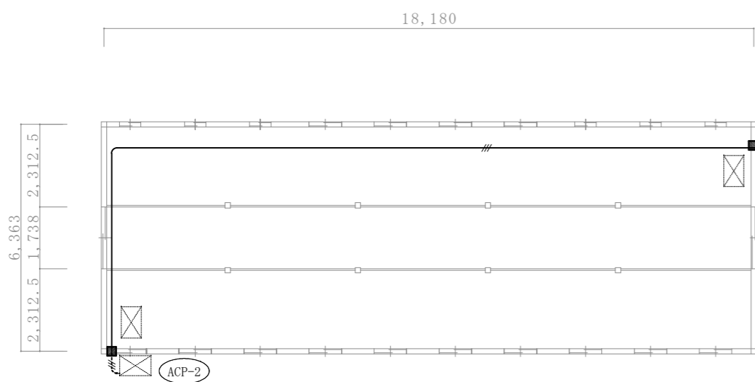
2号廠舎動力設備改修平面図 1:150
