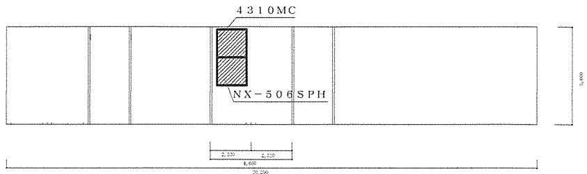
ユニットハウスB平面図
