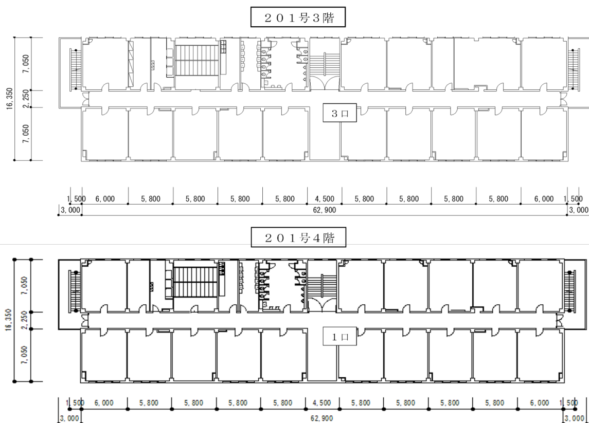
大久保駐屯地コンセント増設配置図
