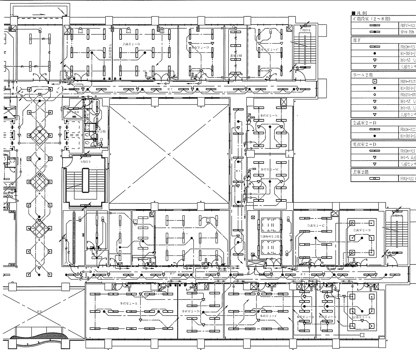
1号建物2階照明器具配置図(東側) S=1/200
