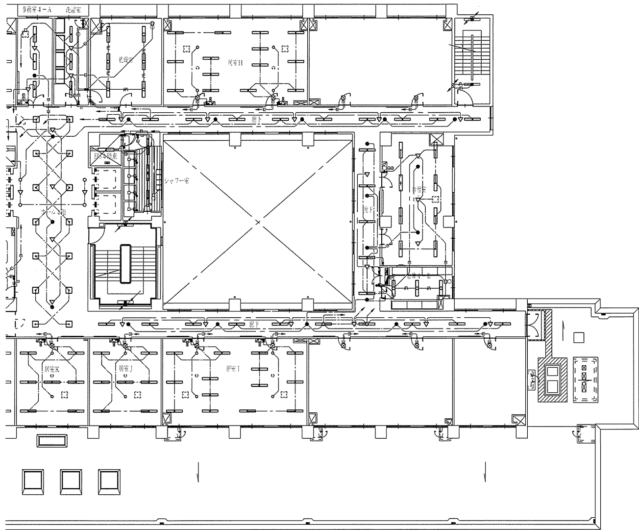
1号建物4階照明器具配置図 (東側) S=1/200
