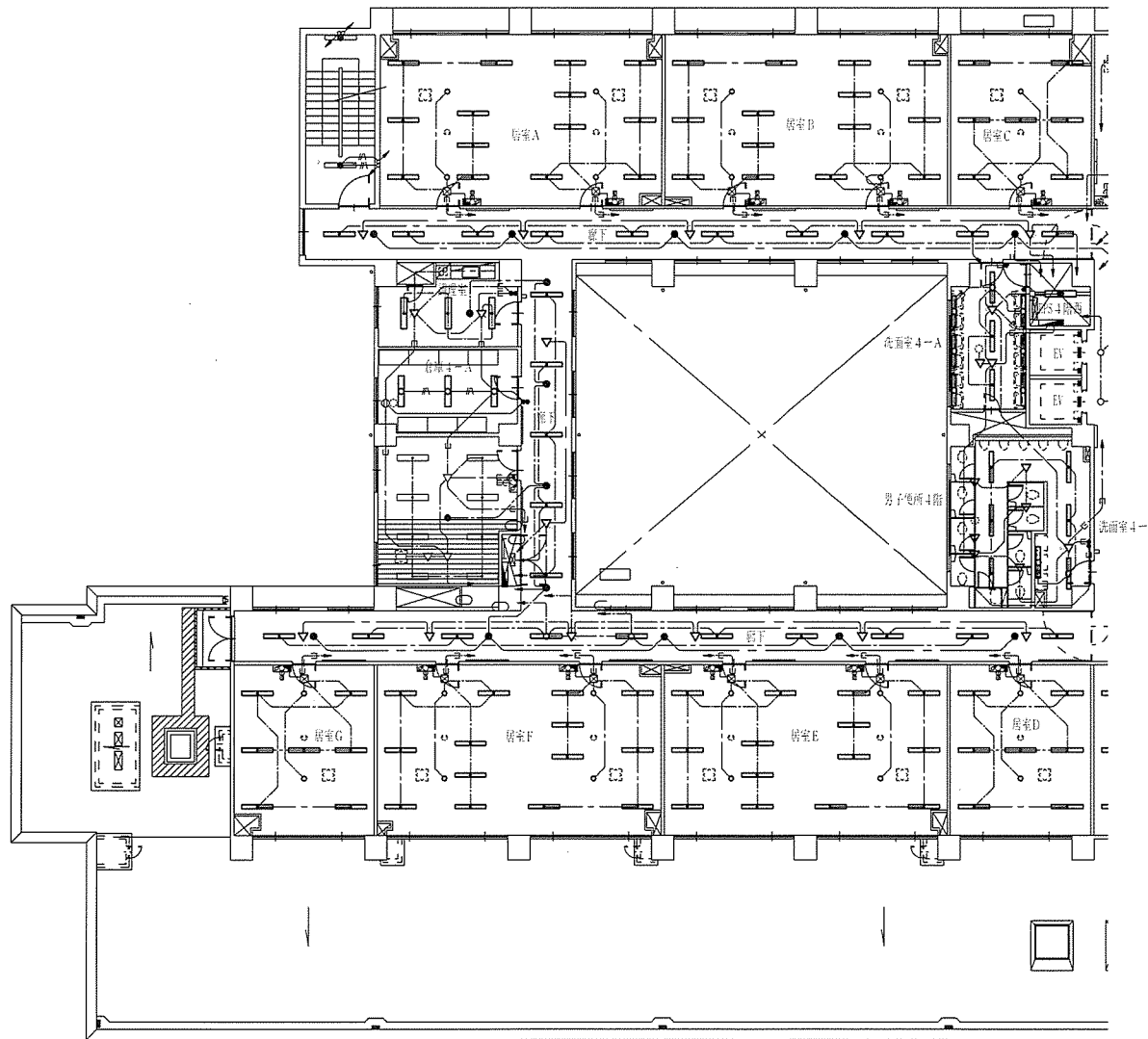
1号建物4階照明器具配置図 (西側) S=1/200
