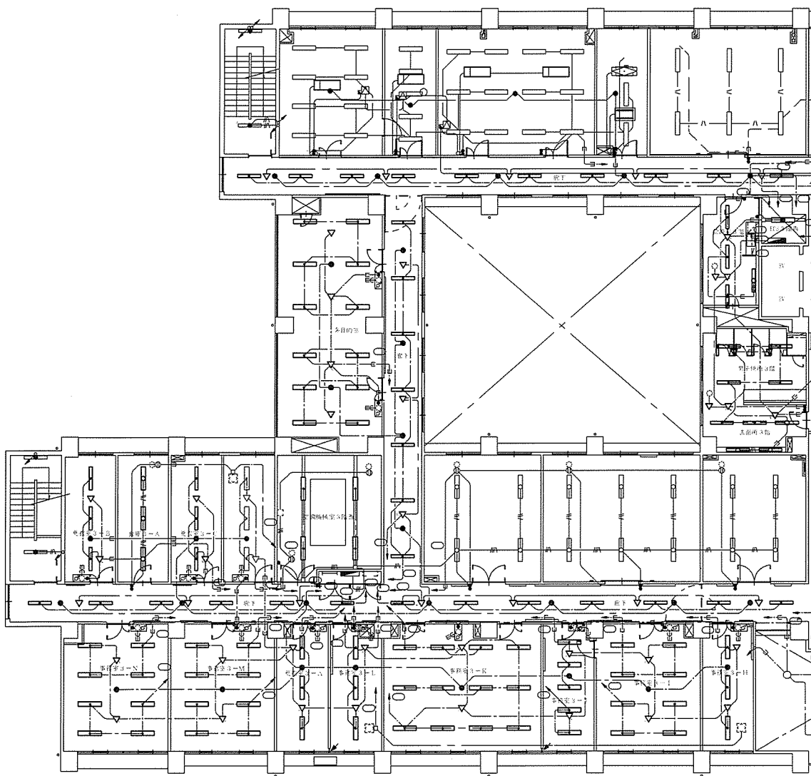
1号建物3階照明器具配置図(西側) S=1/200
