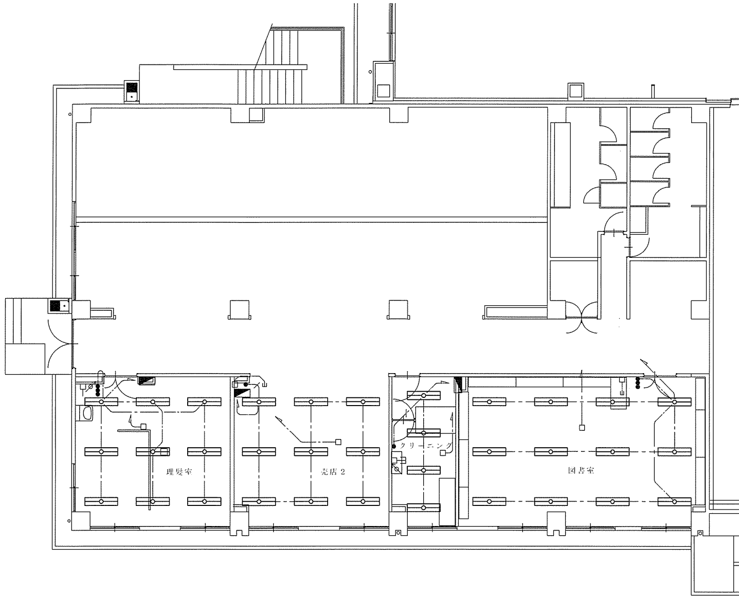
2号建物1階照明器具配置図 S=1/100
