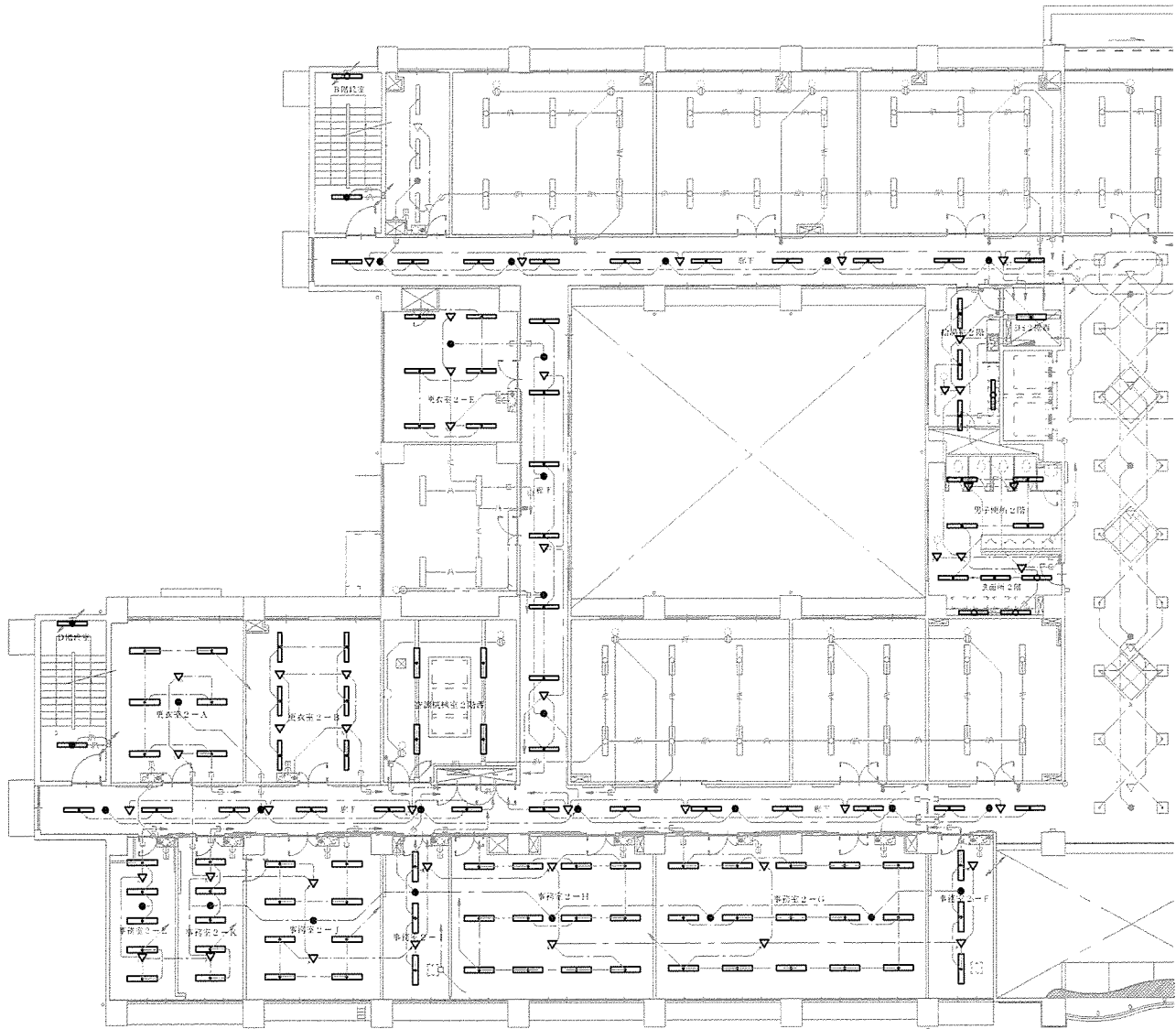
1号建物2階照明器具配置図(西側) S=1/200
