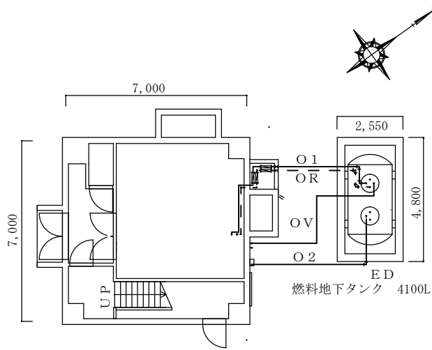
宮路山無線中継所 1階平面図 1/X
