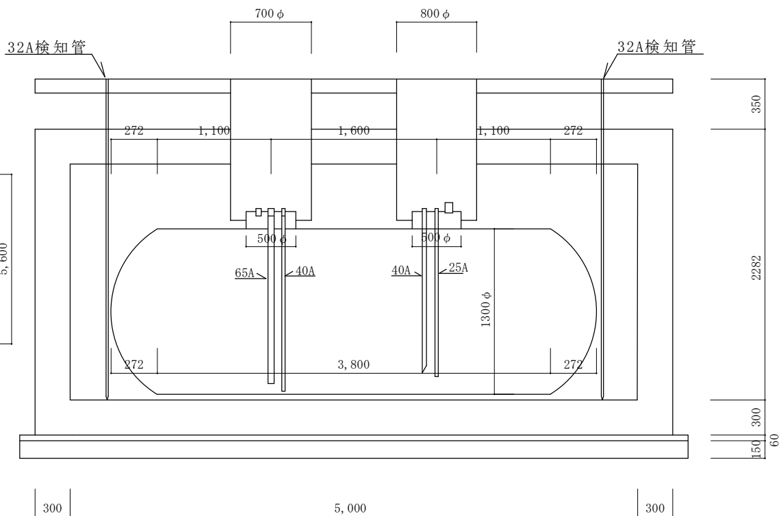
本宮山無線中継所 地下タンク埋設図 1/X
