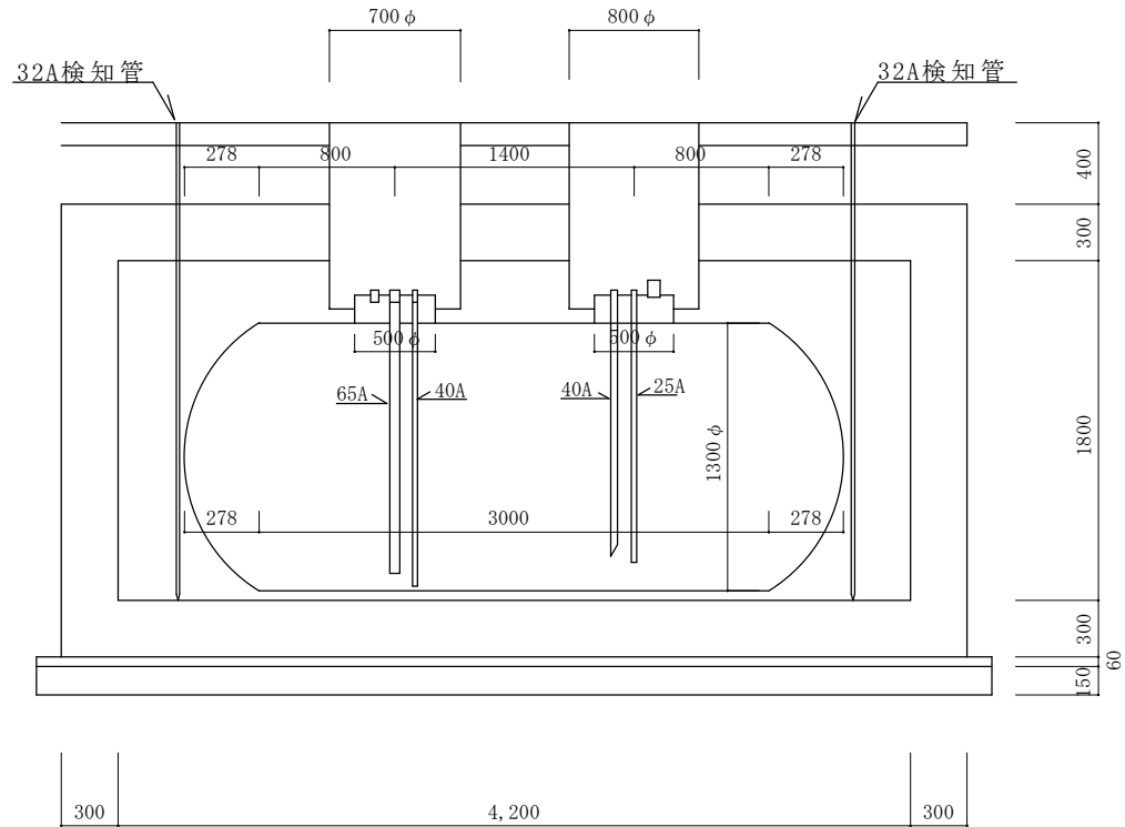
宮路山無線中継所 地下タンク埋設図 1/X
