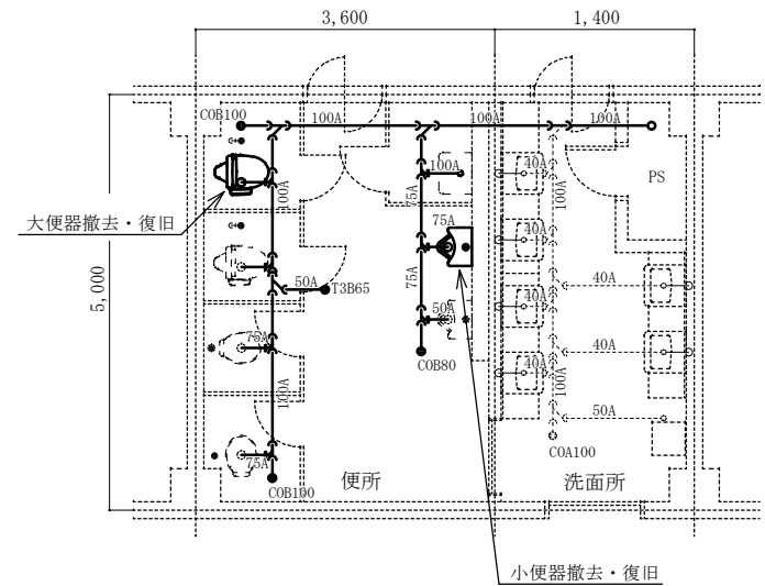
177号建物 2～5階便所・洗面所排水配管詳細図 S=1/100
