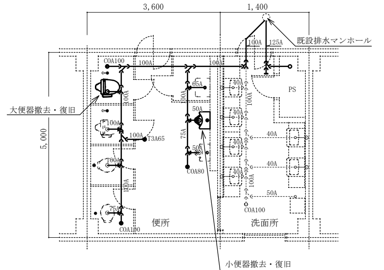
177号建物 1階便所・洗面所排水配管詳細図 S=1/100
