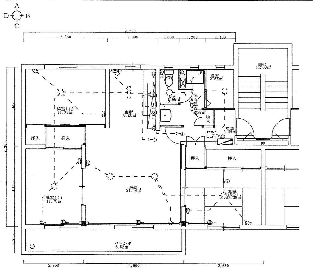
中荒木宿舎 2号棟 (d 規格) 平面図 S=1/100
