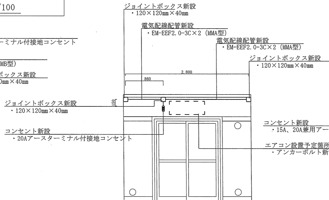
玄関 C面
