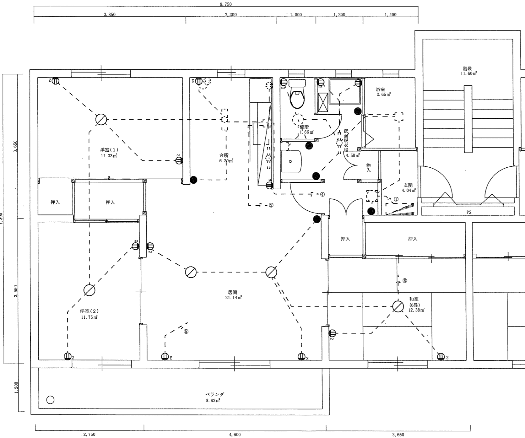
中荒木宿舎 2号棟 (d 規格) 撤去平面図 S=1/60
