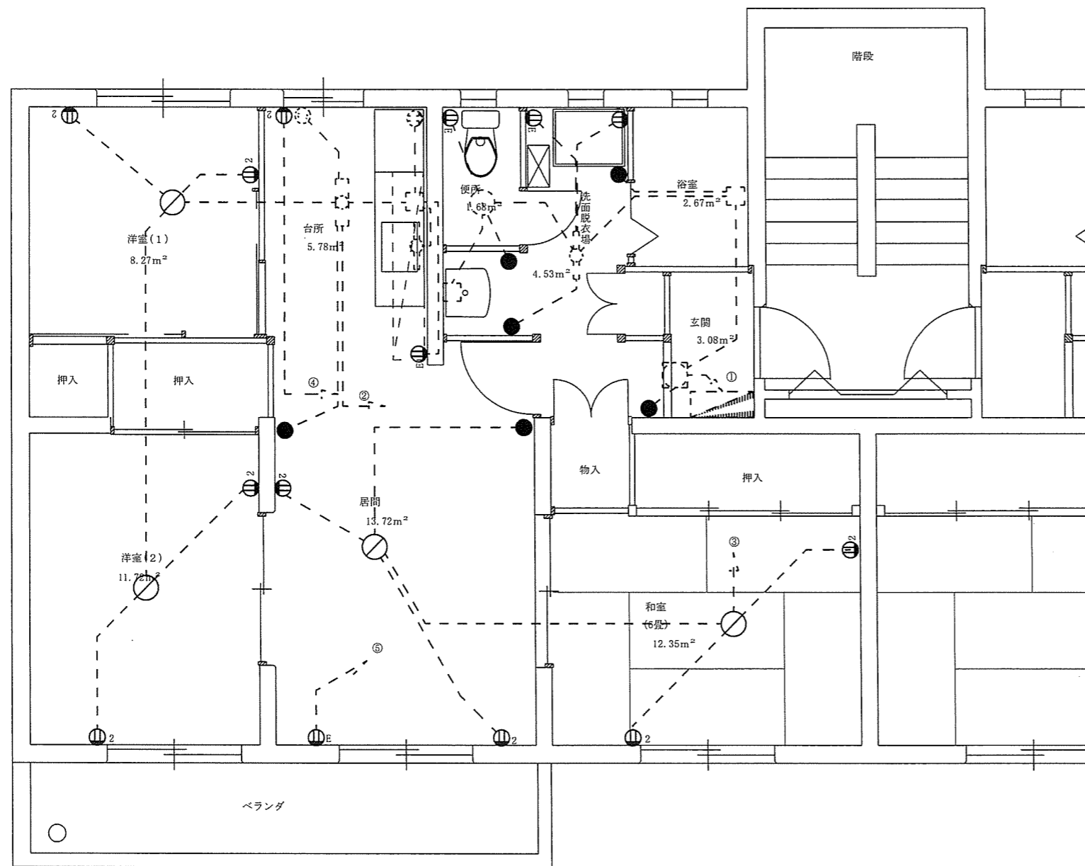
中荒木宿舎 2号棟 (C規格) 撤去平面図 S=1/60
