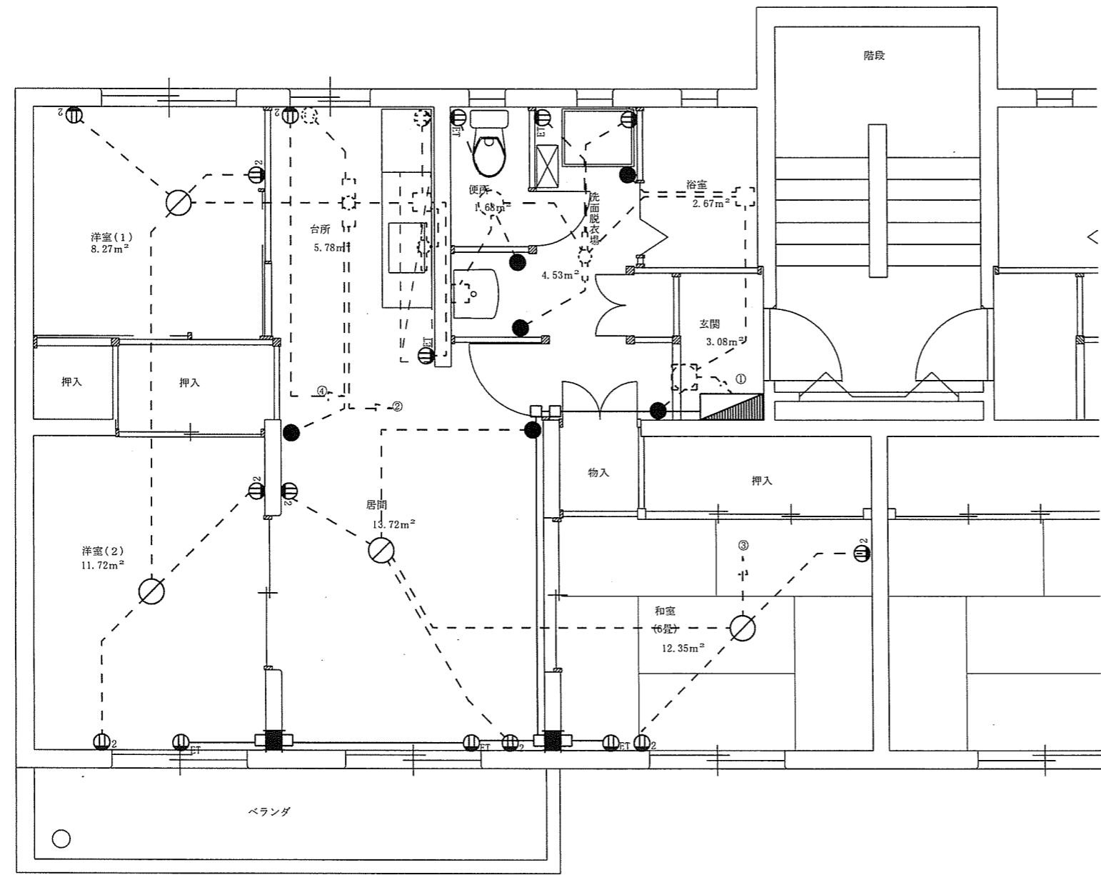
中荒木宿舎 2号棟 (C規格) 新設平面図 S=1/60
