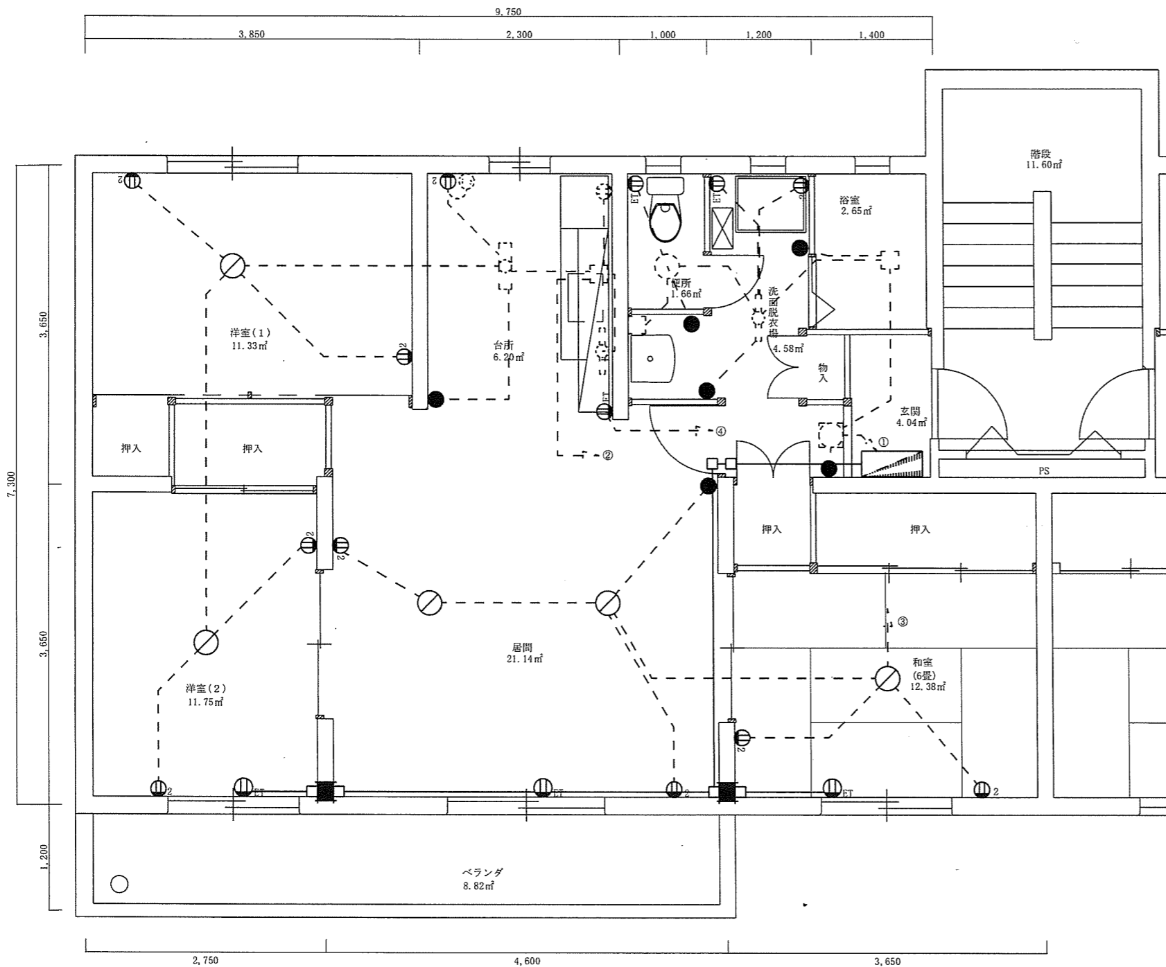
中荒木宿舎 2号棟 (d規格) 新設平面図 S=1/60
