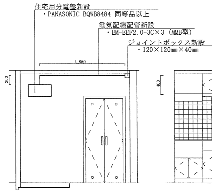
玄関 C面
