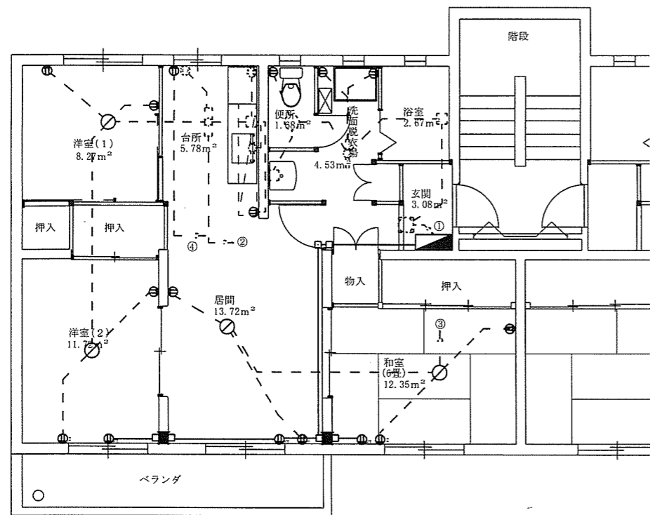
中荒木宿舎 2号棟 (c 規格) 平面図 S=1/100
