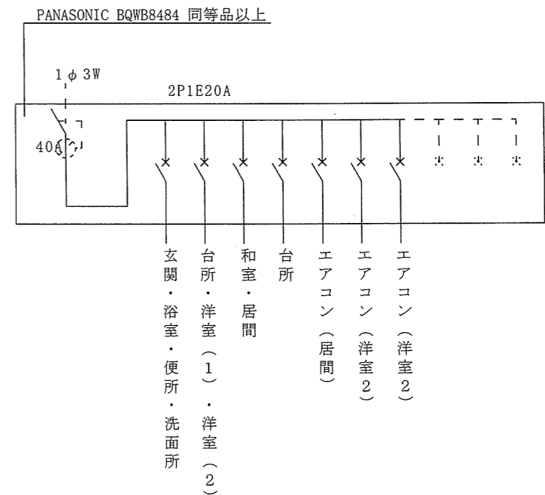
中荒木宿舎 2号棟 (d規格) 分電盤新設詳細図 S=NS
