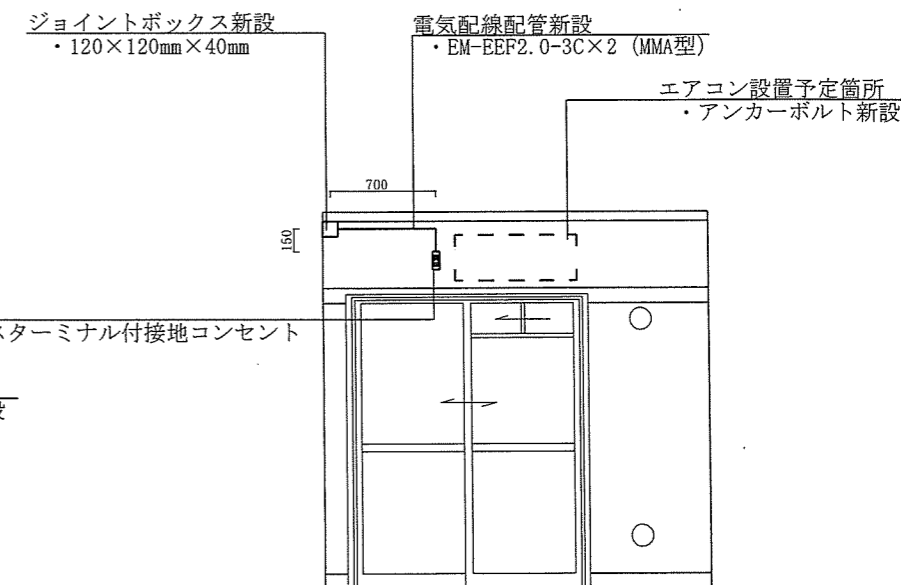
洋室 (2) C面
