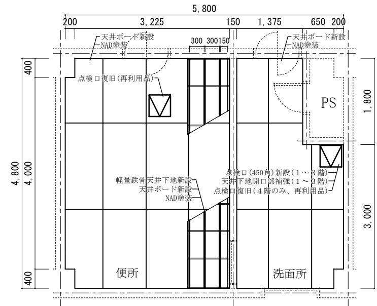
1～4階天井伏図 (改修後)
