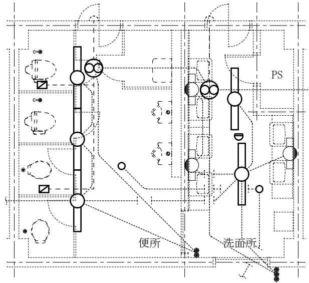
1～4階天井伏図 (改修前)
