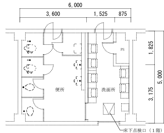
177号建物 1～5階便所・洗面所平面図 S=1/100
