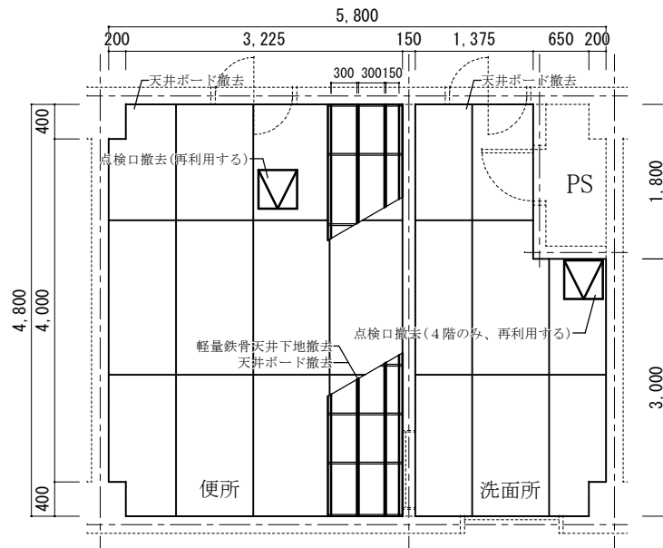
1～4階天井伏図 (改修前)
