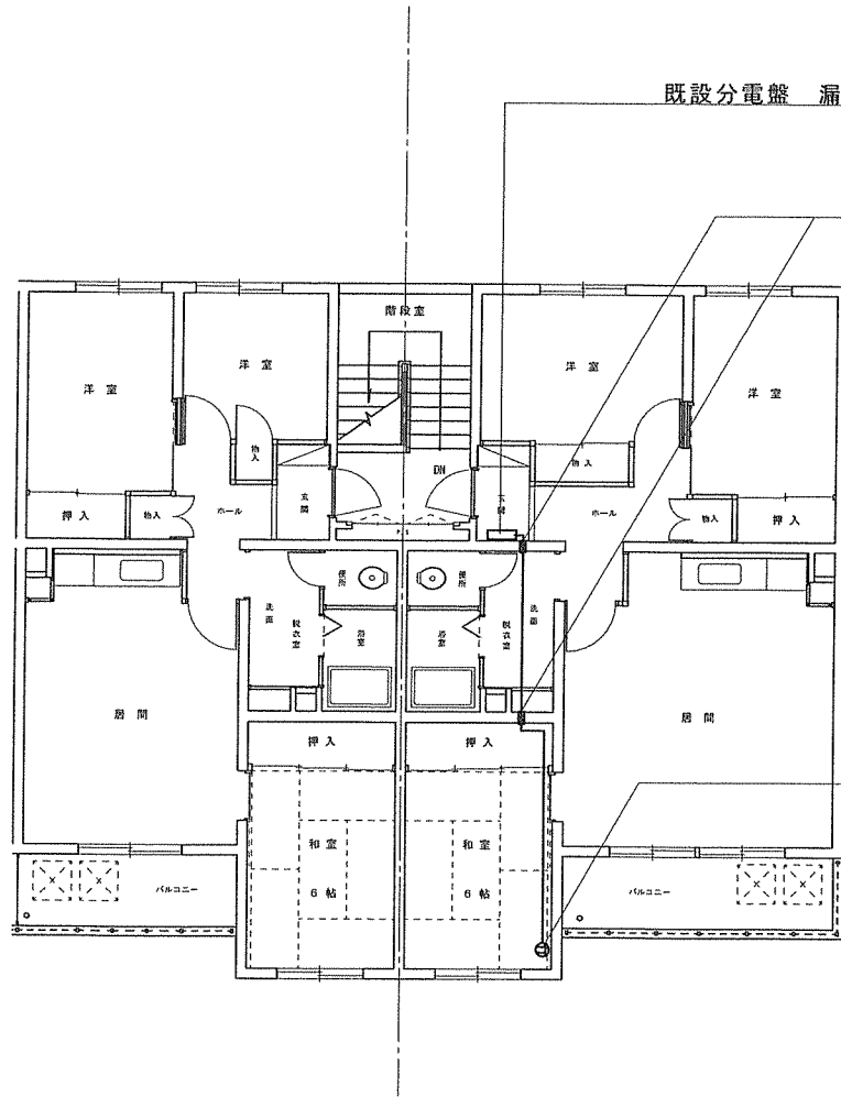
北梅本宿舎1号棟平面図 S=1/100
