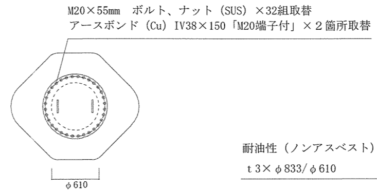
側面マンホール 立面図① S = 1 / 5 0
