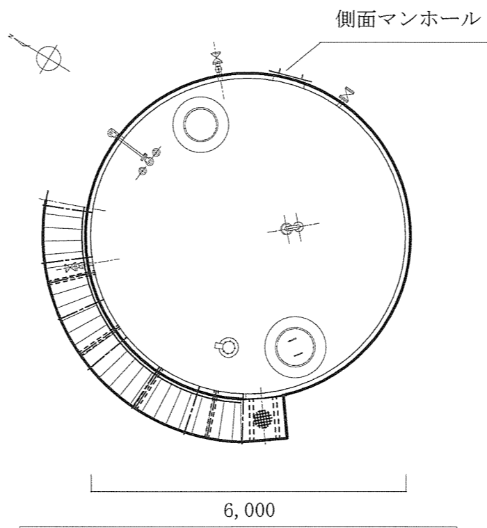
屋外タンク 平面図 S = 1 / 1 0 0
