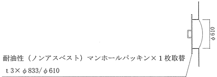
側面マンホール 立面図② S = 1 / 5 0
