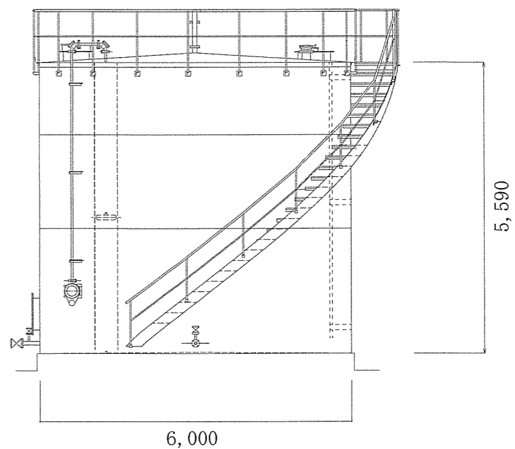
屋外タンク 西面立面図 S = 1 / 1 0 0
