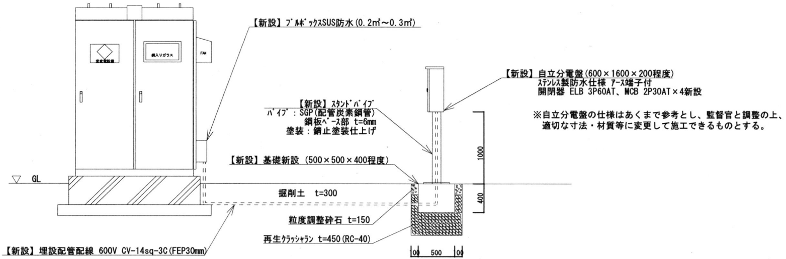
立面図 (施工場所②)
