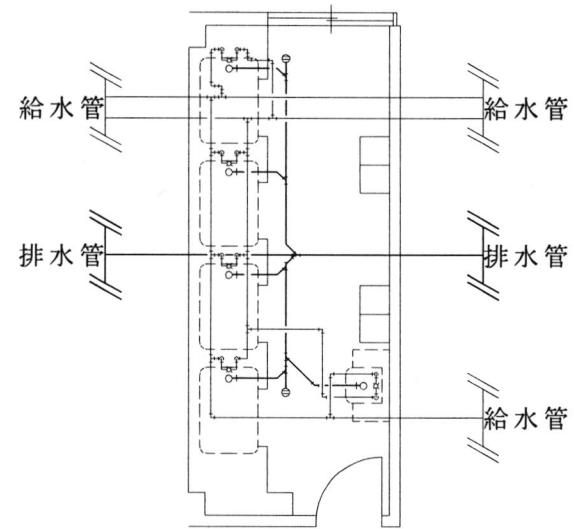
給水設備図 S=1:100
