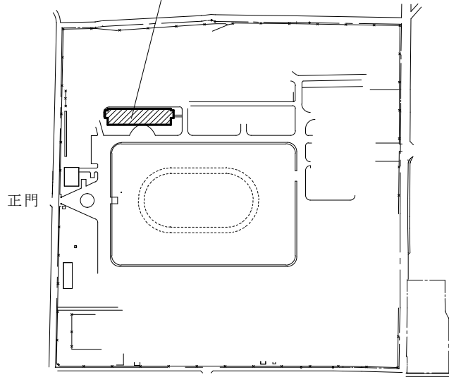
配置図 1:4,000
