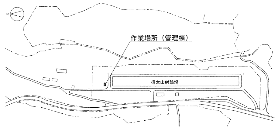
演習場配置図 S=1/6,000
