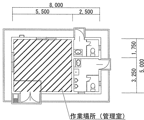
管理棟平面図 S=1/200
