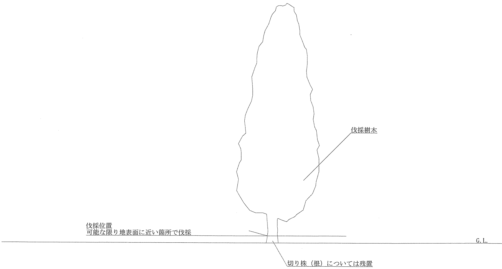
樹木伐採要領詳細図 S=1/25
