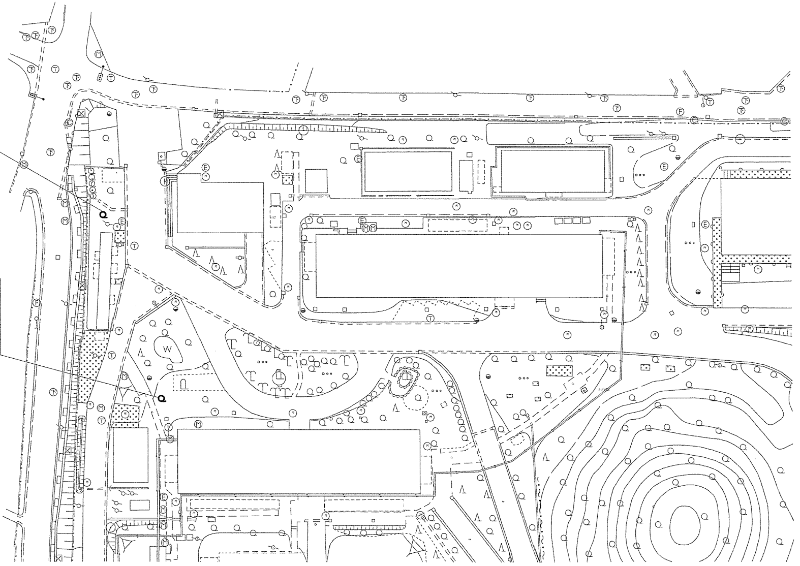
作業場所A詳細図 S=1/400
