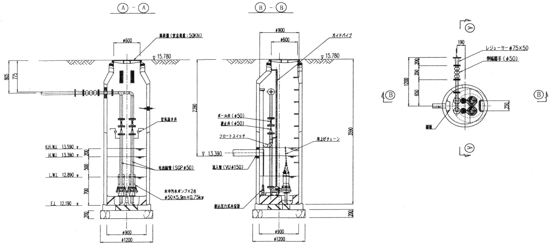
汚水中継槽詳細図 S = 1 / X
