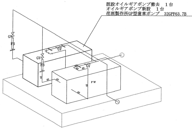
ポンプ室内配管詳細図 S=1/40
