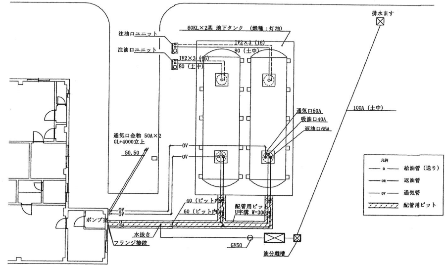
配管系統図 S=1/300
