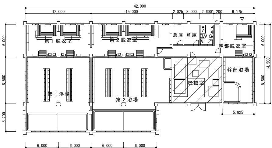
浴場平面図 S = 1/300
