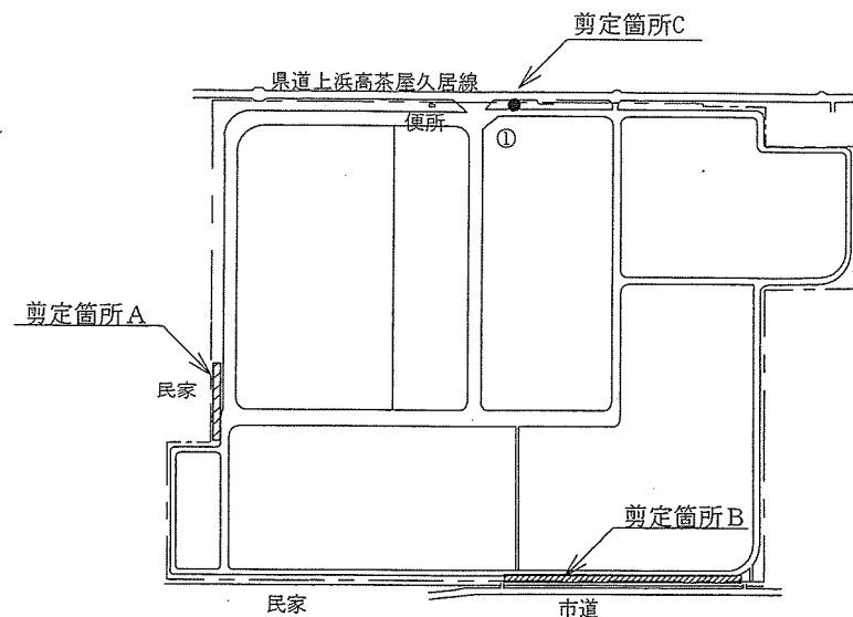
久居訓練場配置図 1 : X
