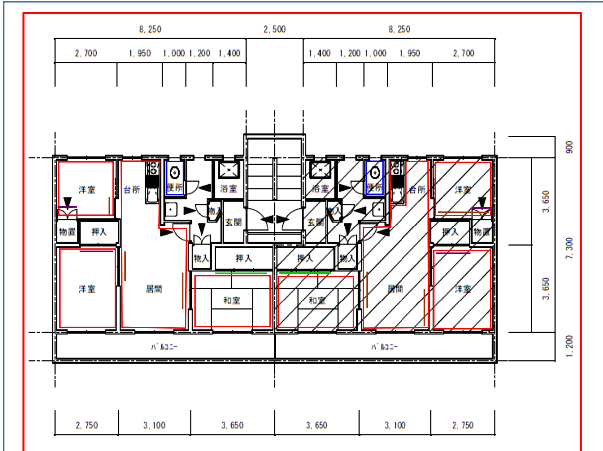
301・302号室平面詳細図（基準階）
