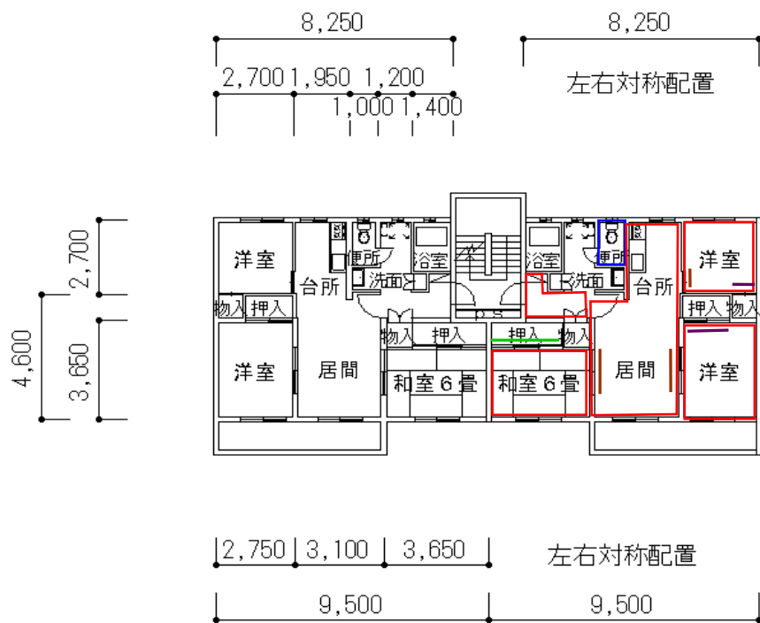
2～9号室平面詳細図 (基準階)
