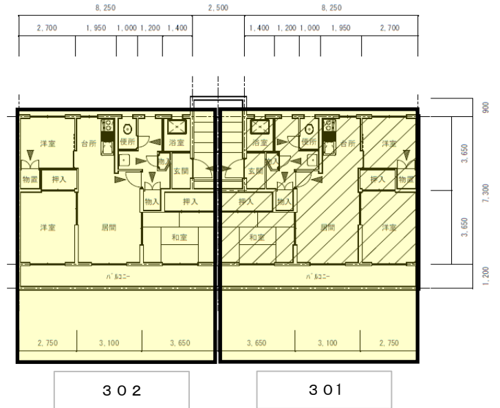
浜坂宿舎平面図（基準階）
