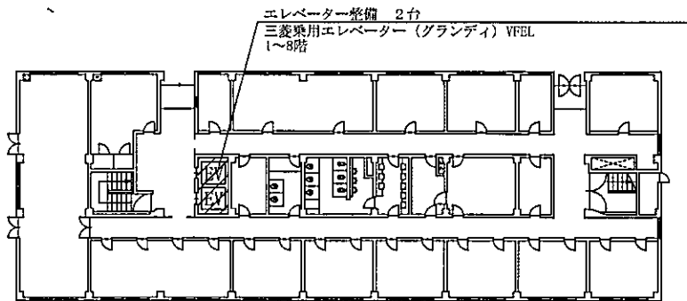
271号建物平面図 S=1/400
