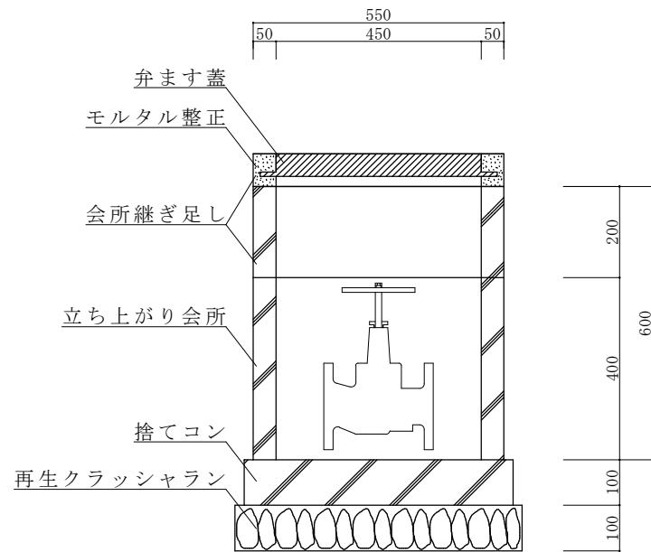
弁枒②詳細図 S = 1 : 1 0
