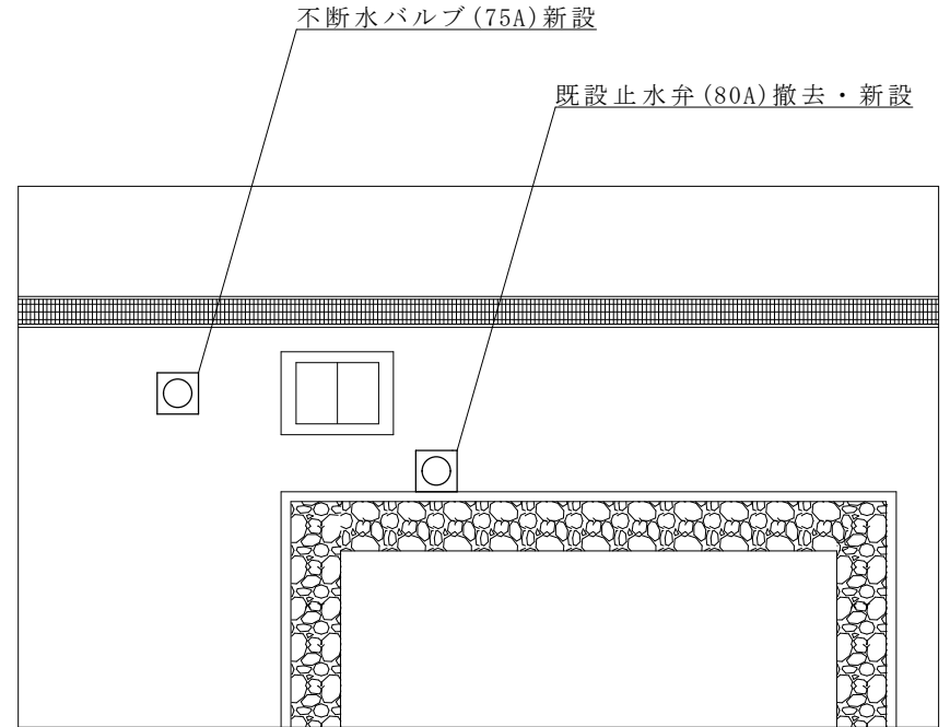
工事実施場所詳細平面図 S = 1 : 1 0 0
