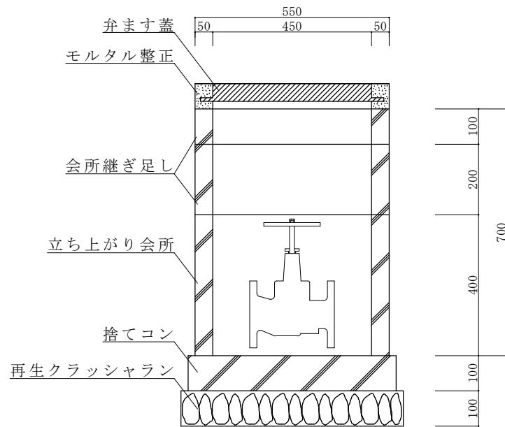
弁枒①詳細図 S = 1 : 1 0
