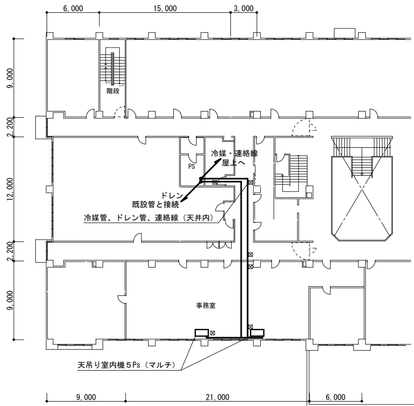
2階平面図 S=1/300
