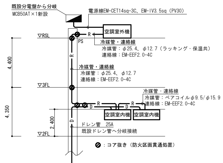
幹線・配管系統図 S=1/150
