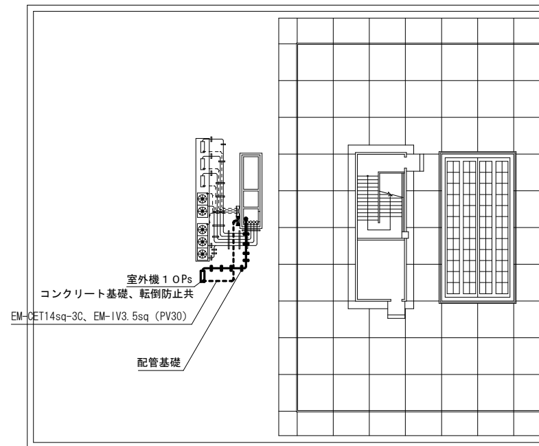
屋上平面図 S=1/300
