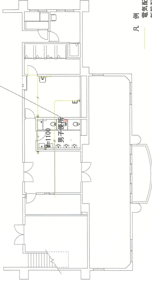
体育館2F 電気 (コンセント) 平面図 1/200
