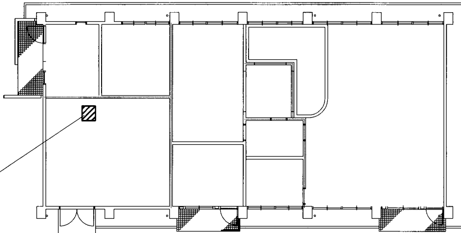
119号浴場平面図 S=1/200
