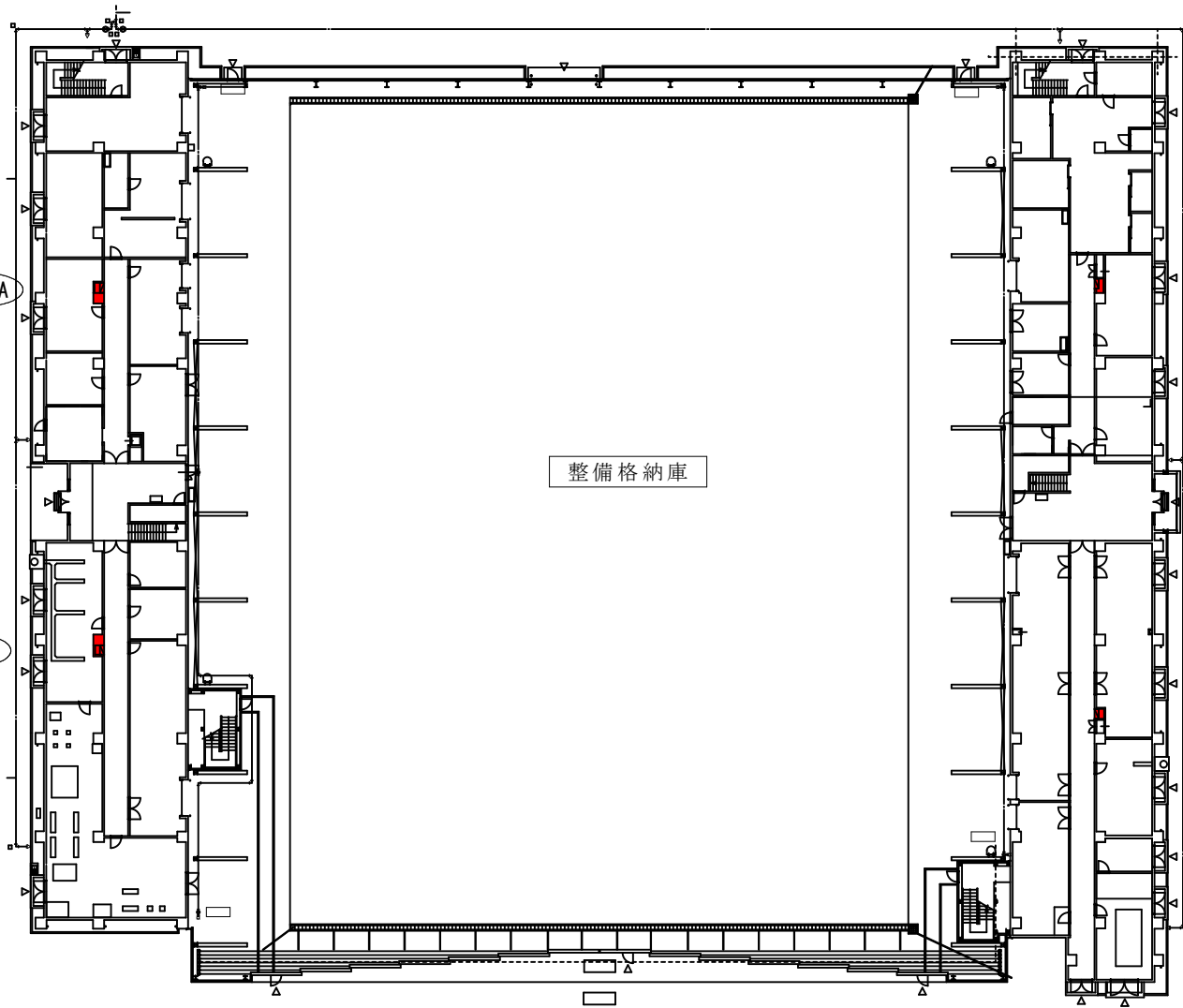
格納庫内 1F 屋内消火栓設備配置図 S=1/600
