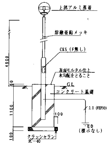
277号廻り外灯立面図
