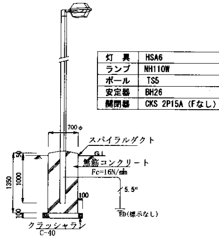
268号廻り外灯立面図
