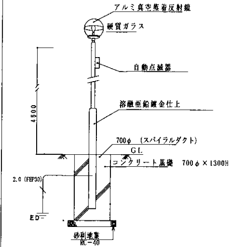
276号廻り外灯立面図
