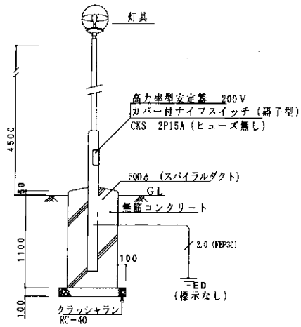
248号廻り外灯立面図
