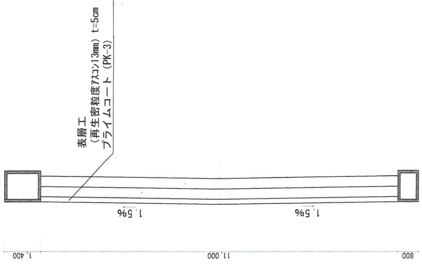
アスファルト舗装断面図
