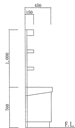
洗面台詳細図 (側面) S=1/40
