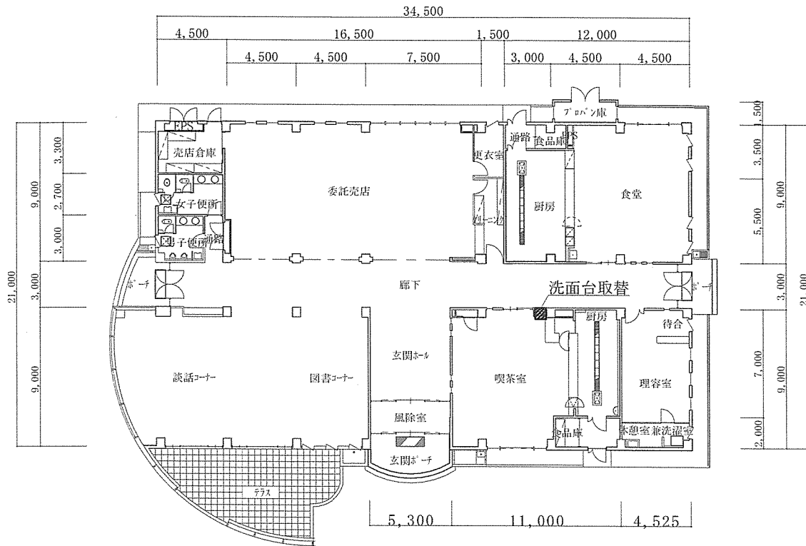
169号建物平面図 S=1/400
