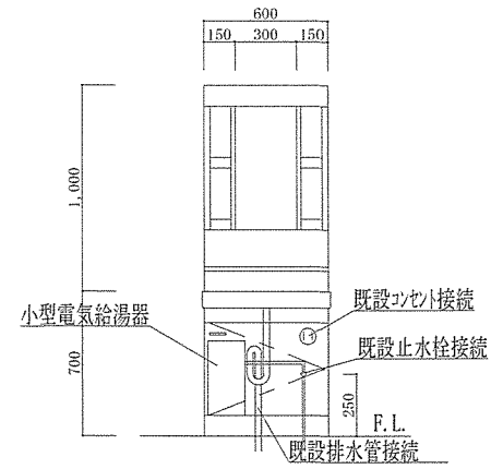
洗面台詳細図 (正面) S=1/40
