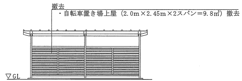
自転車置き場立面図
