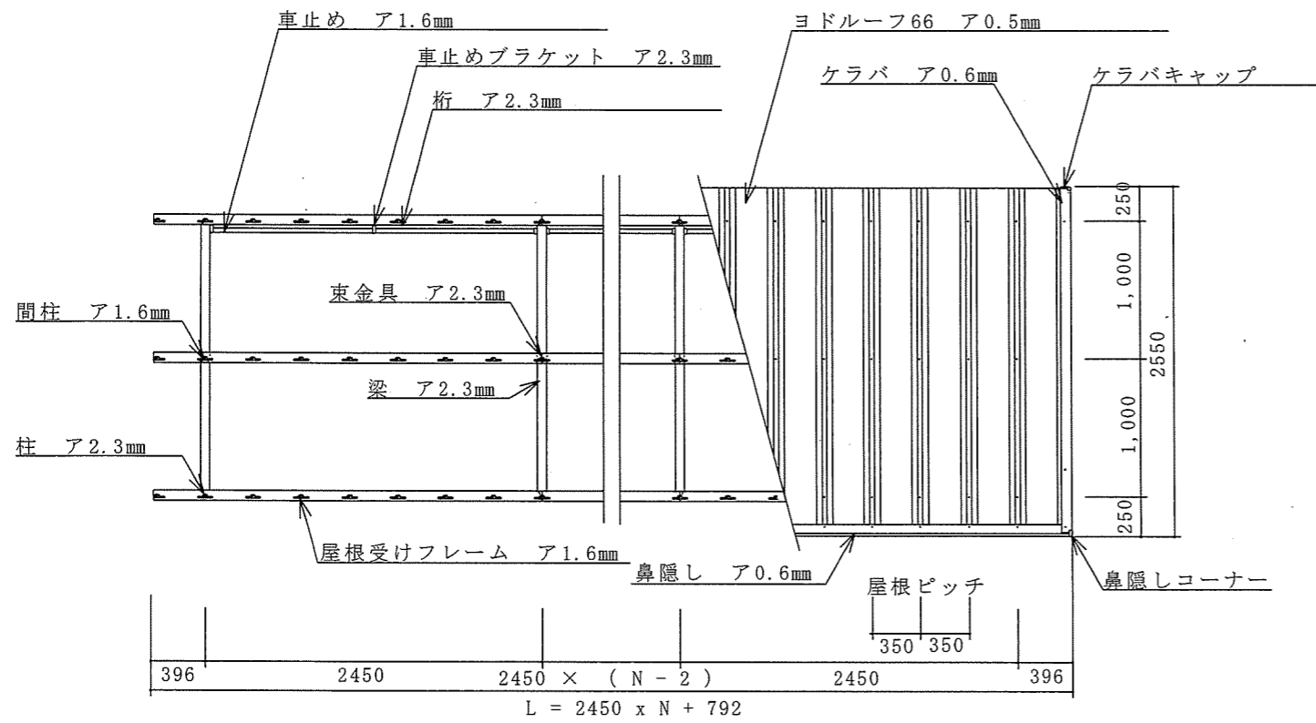
自転車置き場立面図
