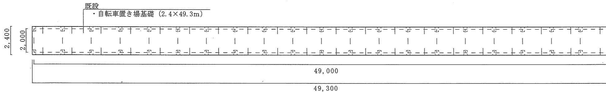
自転車置き場基礎平面図
