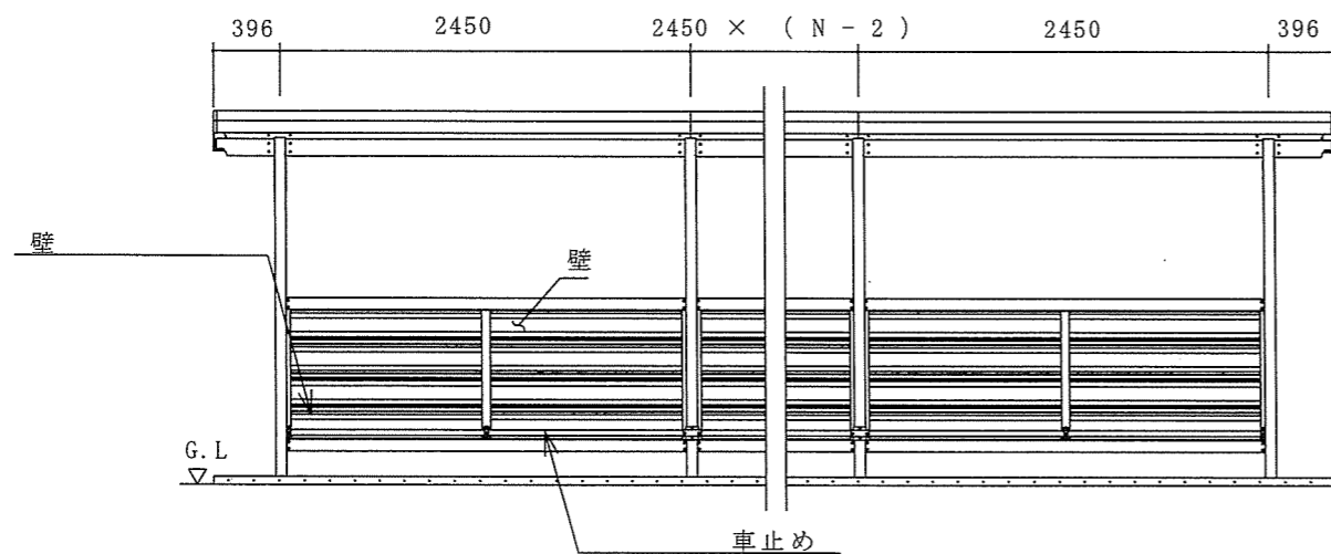
正面立面図
