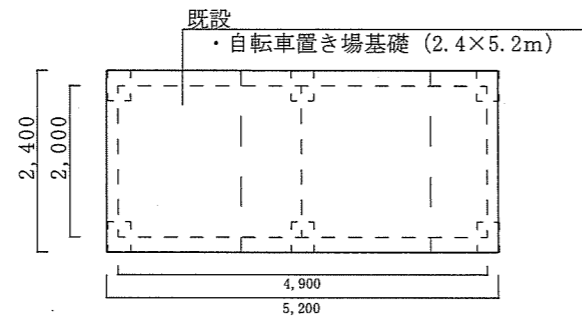
自転車置き場基礎平面図
