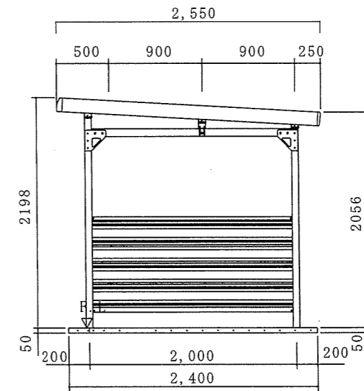
側面立面図
