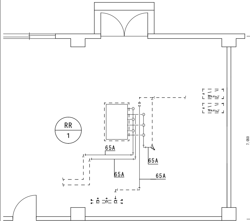
61号建物機械室平面図 S=1:100
