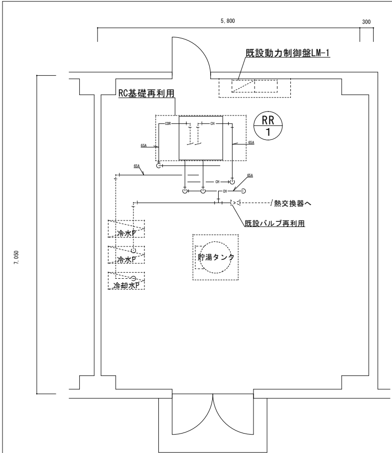
61号建物機械室平面図 S = 1 : 100
