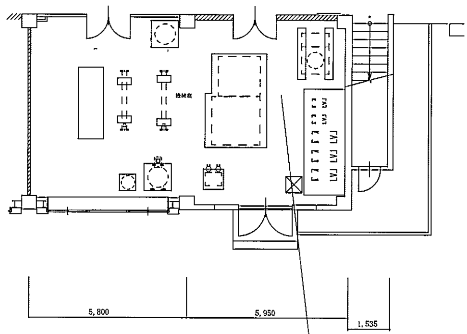
平面図 S=1/150
