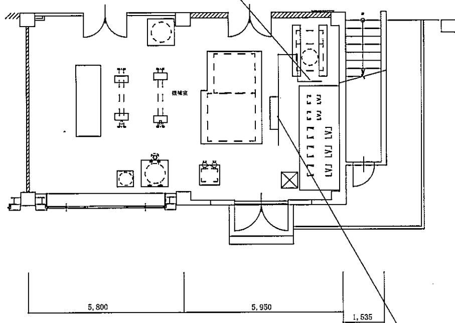
平面図 S=1/150
