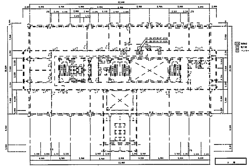
290号建物2階平面図 S=1/400
