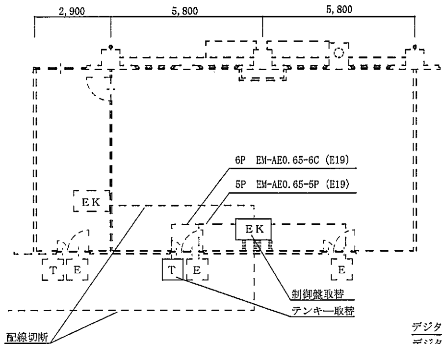
既設290号建物2階平面図 S=1/400
