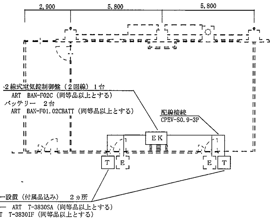
既設290号建物2階平面図 S=1/400
