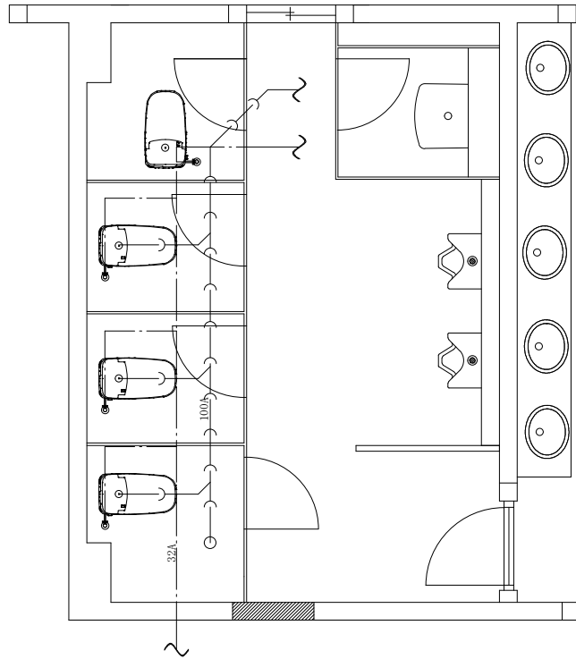
234号5階便所改修前給排水配管図 S = 1 : 40
