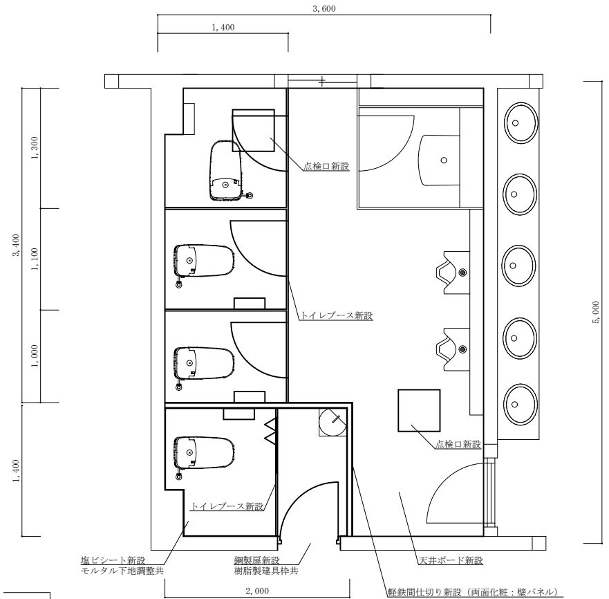
234号5階便所改修後平面図 S=1:40
