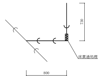
便所排水管アイソメ図 S = 1 : 30
