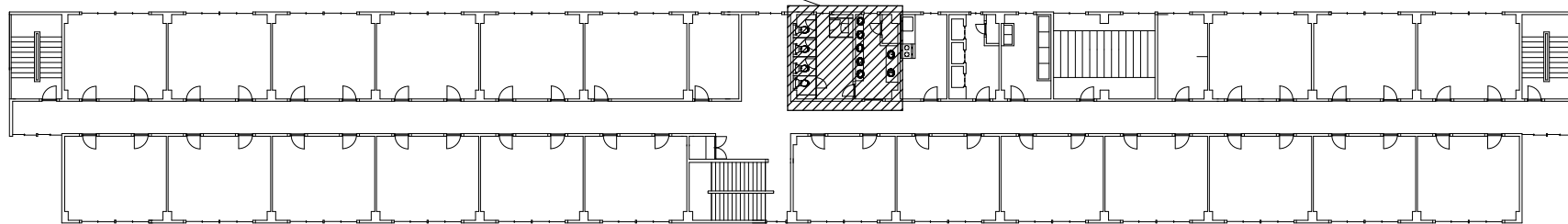
234号建物5階平面図 S = 1 : 4 0 0
