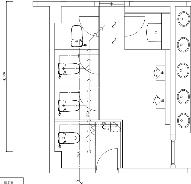
234号5階便所改修後給排水配管図 S = 1 : 40
