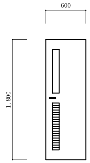
新設鋼製扉詳細図 S=1:40
