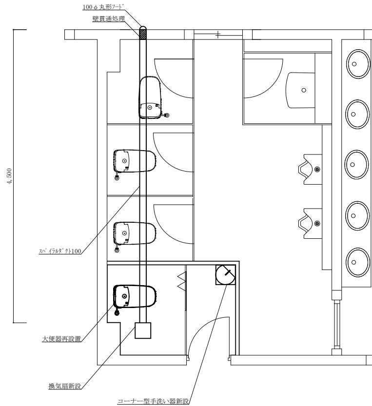
234号5階便所改修後衛生・換気設備平面図 S = 1 : 40
