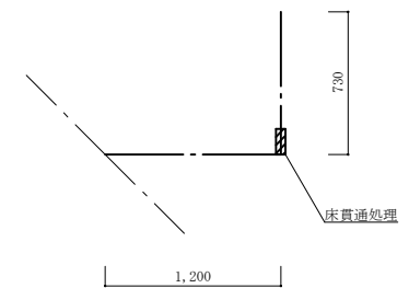
便所給水管アイソメ図 S = 1 : 30
