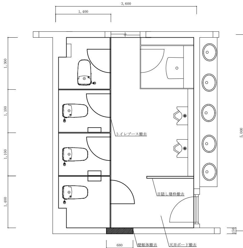
234号5階便所改修前平面図 S=1:40
