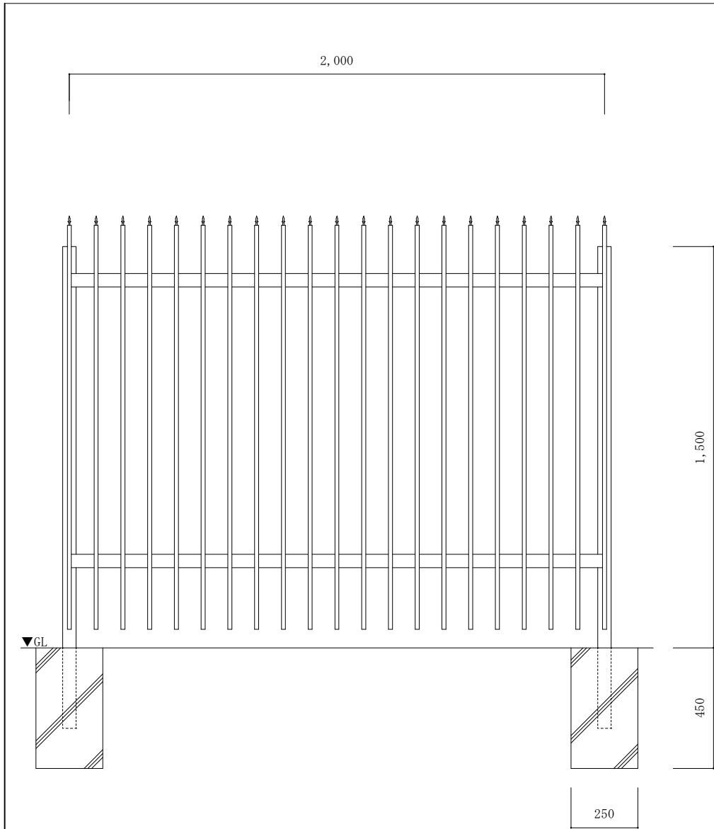
既存外柵詳細図 S = 1 : 20
