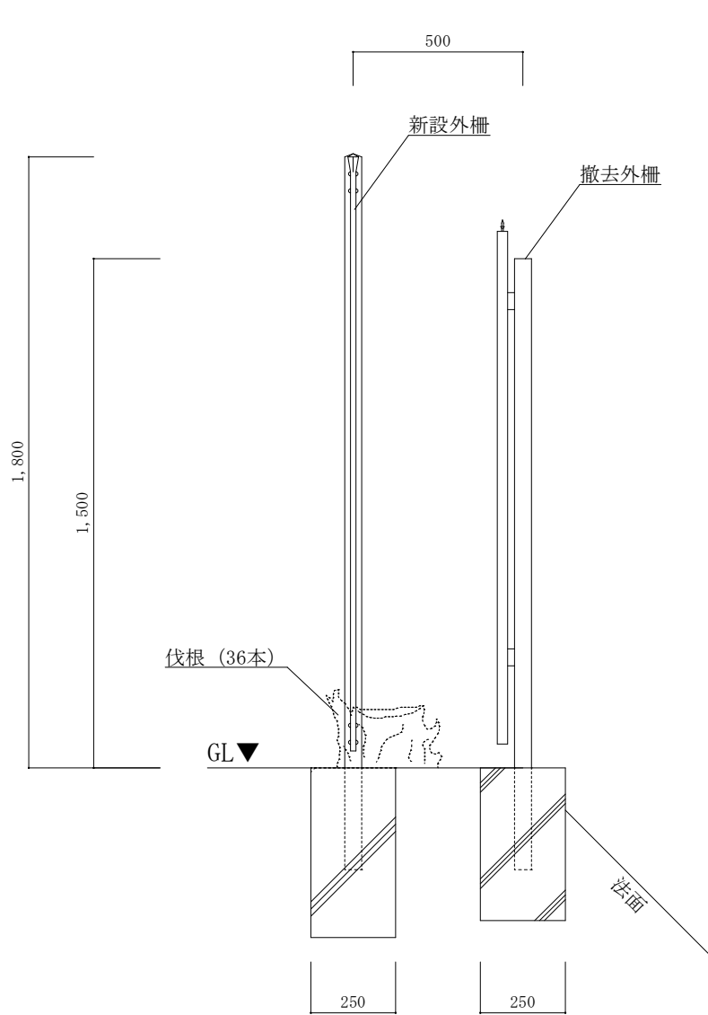
外柵立面図 (側面) S = 1 : 20
