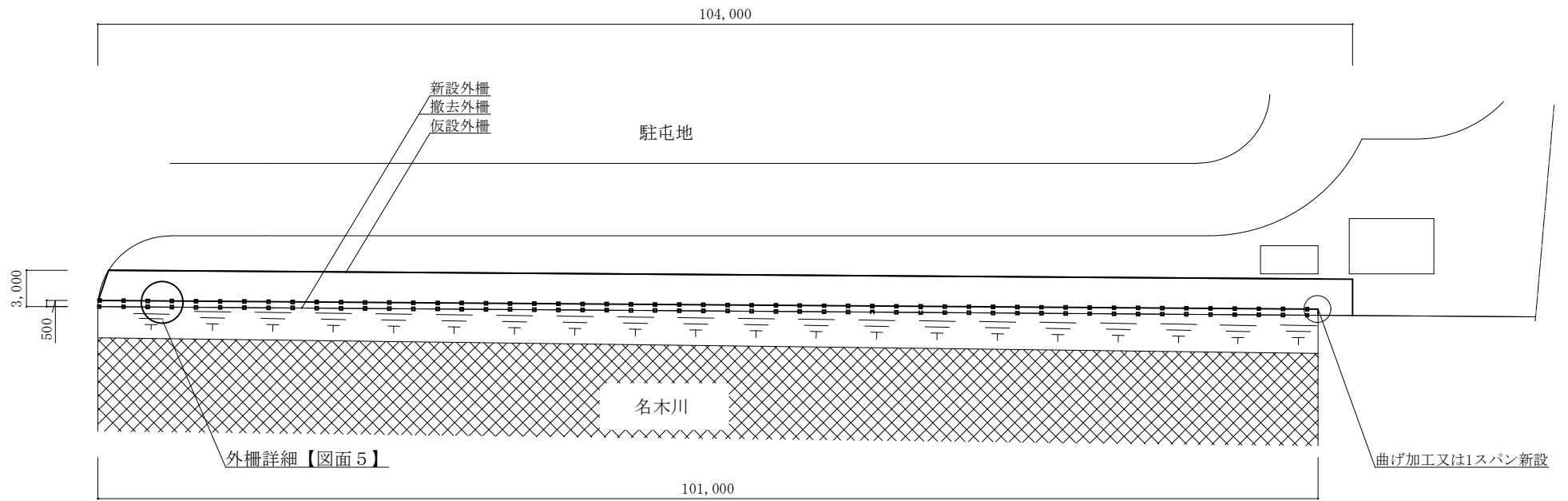
外柵配置図 (改修) S = 1 : 500
