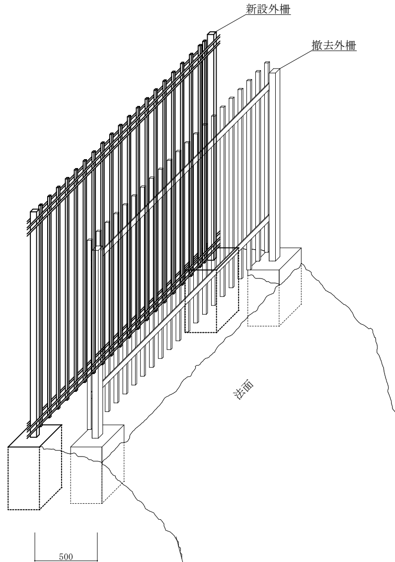
外柵立体図 S = 1 : 30
