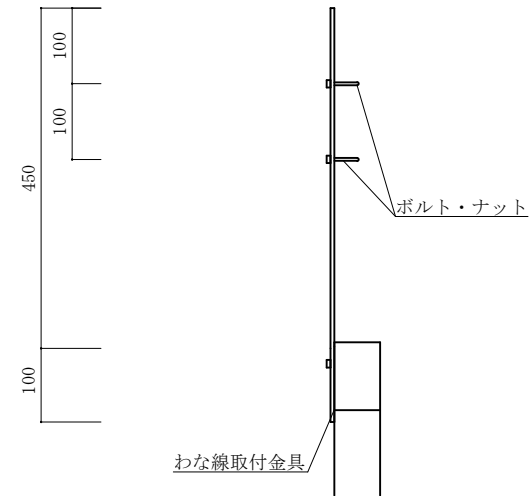
わな線取付金具詳細図 S = 1 : 10
