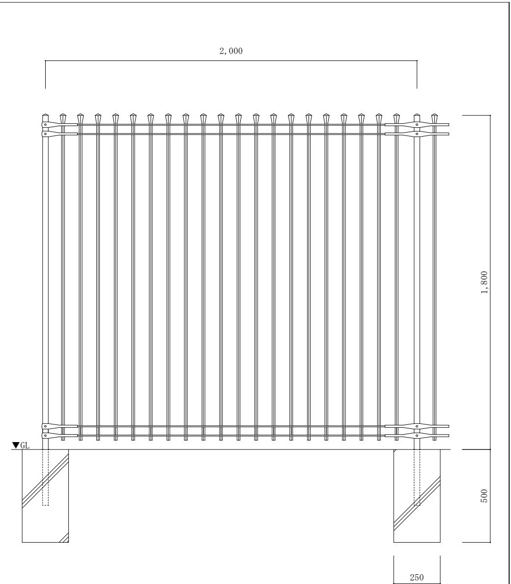
新設外柵詳細図 S = 1 : 20
