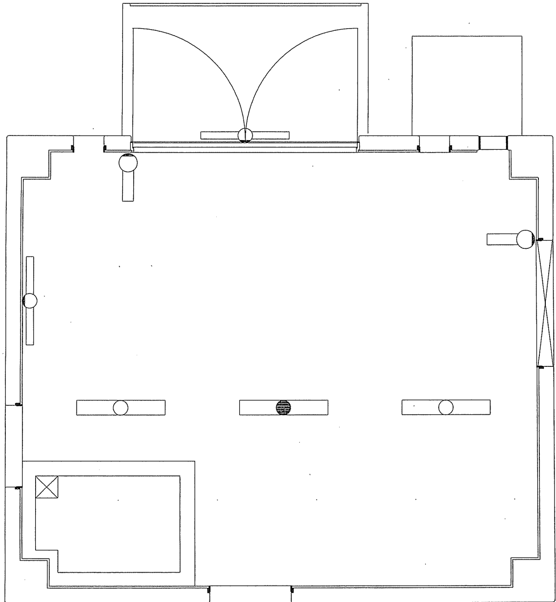
予備発電室照明設備平面図
