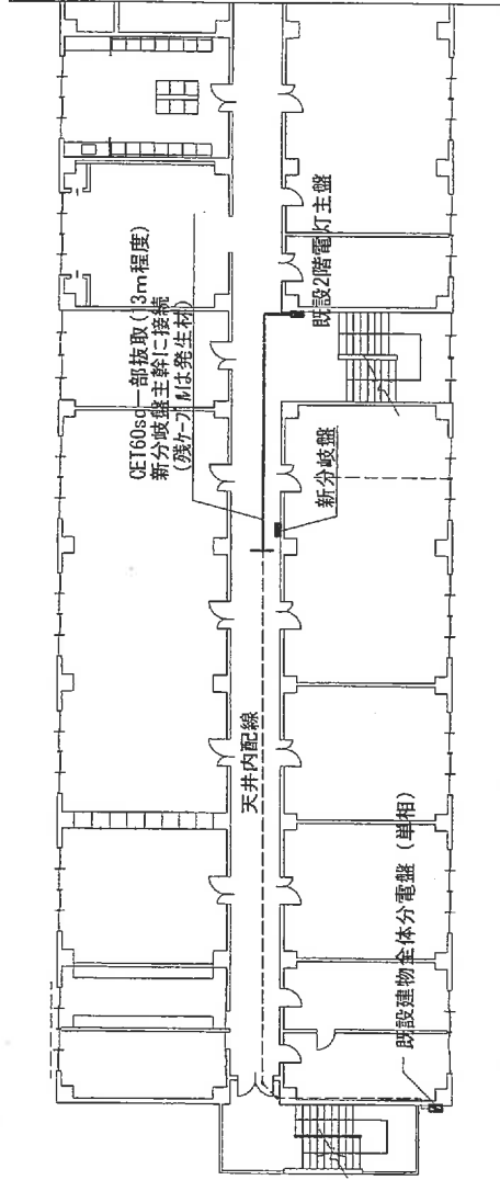
2階平面図 (既設ケーブル撤去図) S=1:350
