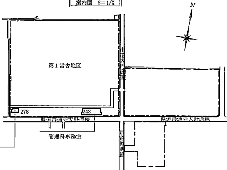
普通寺駐屯地配置図 S=1/5,000
