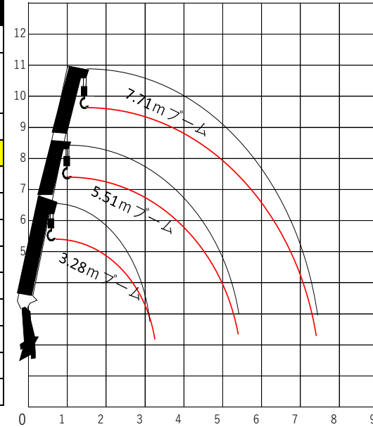
作業半径-揚程図
