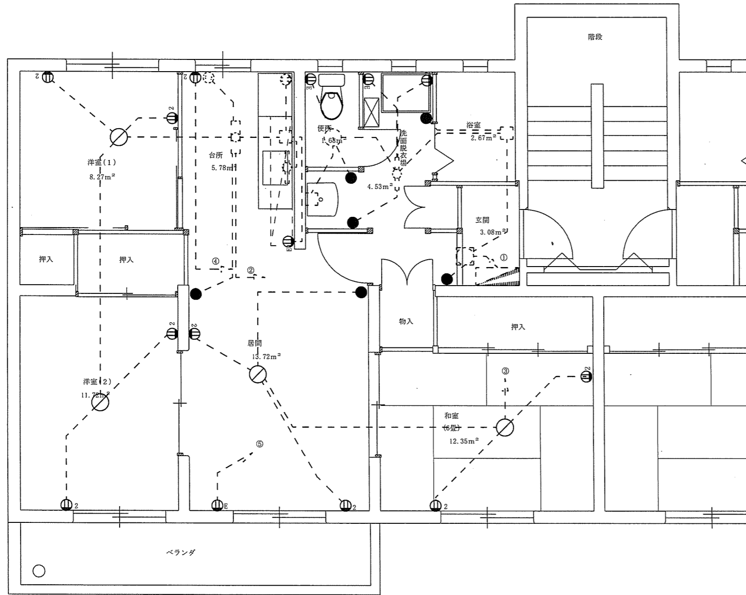
中荒木宿舎 2号棟 (C規格) 撤去平面図 S=1/60
