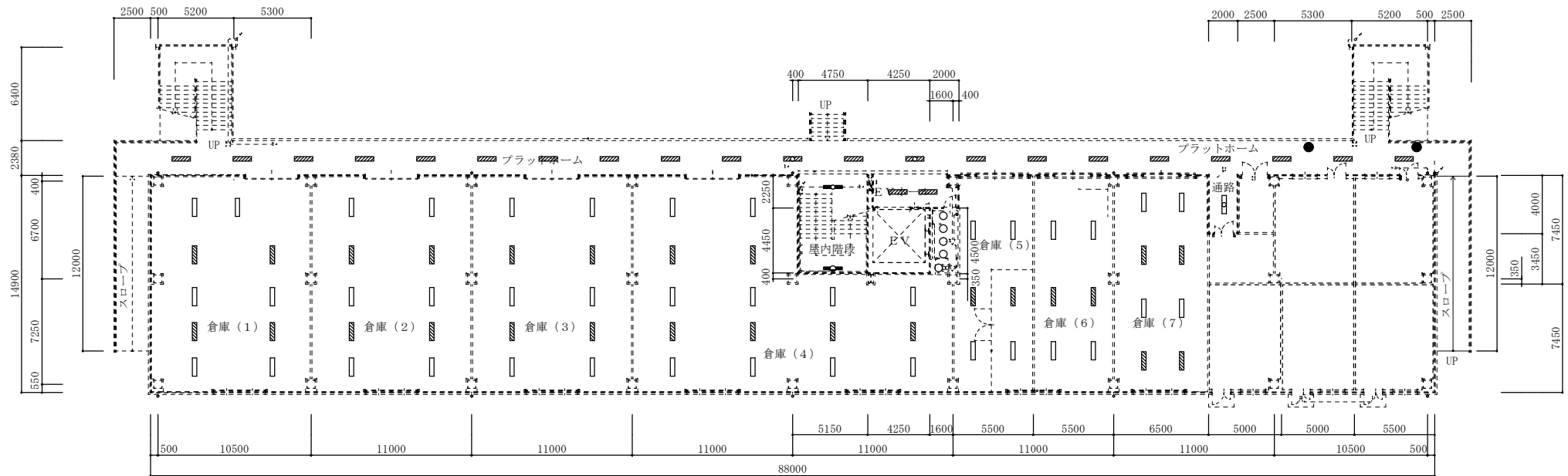
1階平面図
