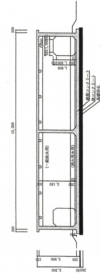
B-B断面 S=1/120
