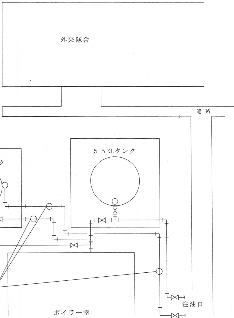
ボイラー埋設管平面図 S : 1 / 200
