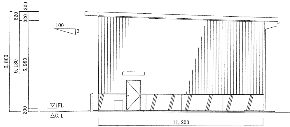
139号建物立面図（改修前） S=1/150
