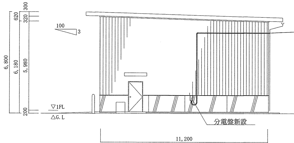
139号建物立面図（改修後） S=1/150
