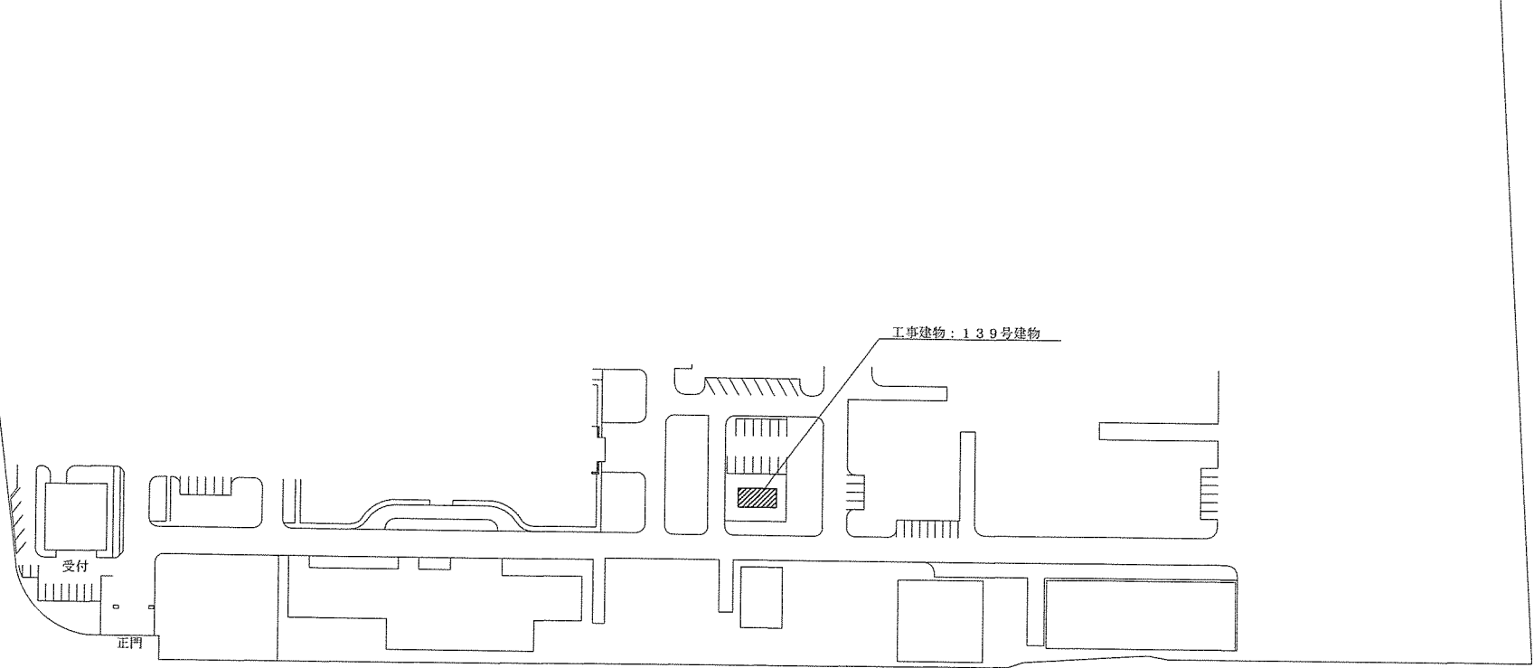
守山駐屯地配置図 S=1/2,000
