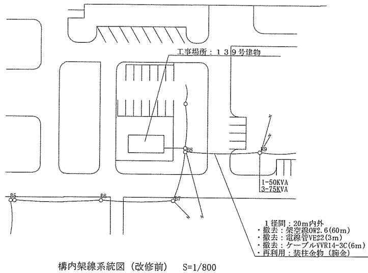
構内架線系統図 (改修前) S=1/800
