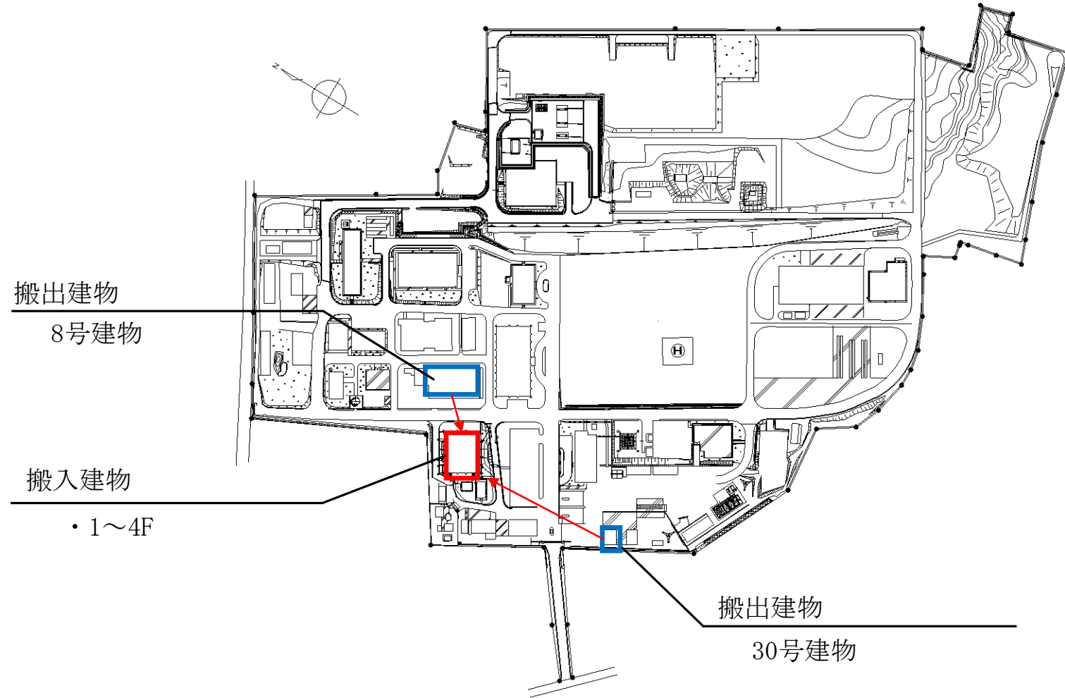
配置図 S=1/4,000
