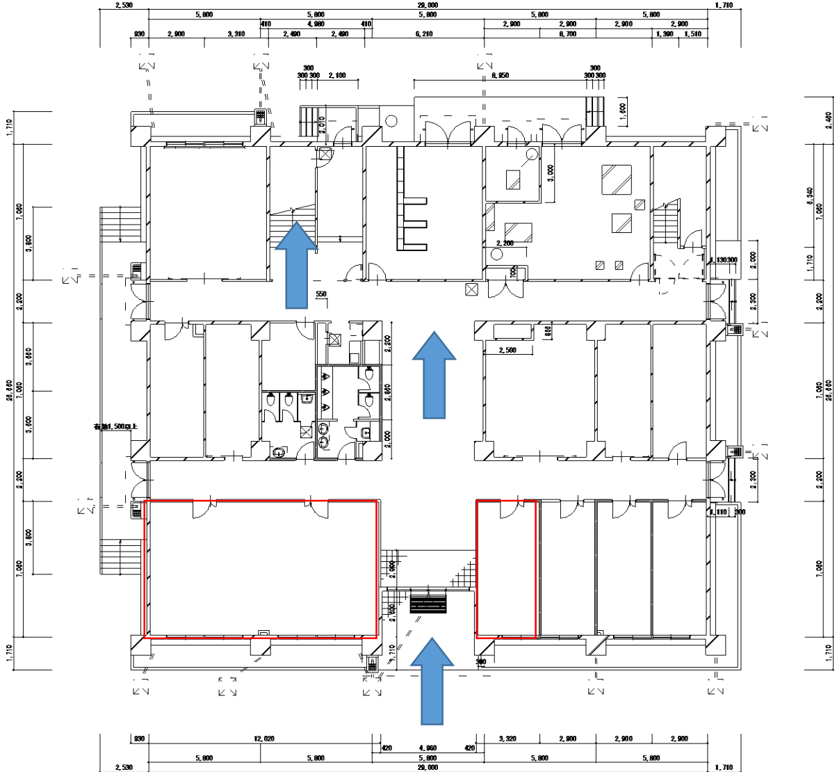
図2－新隊舎1F
