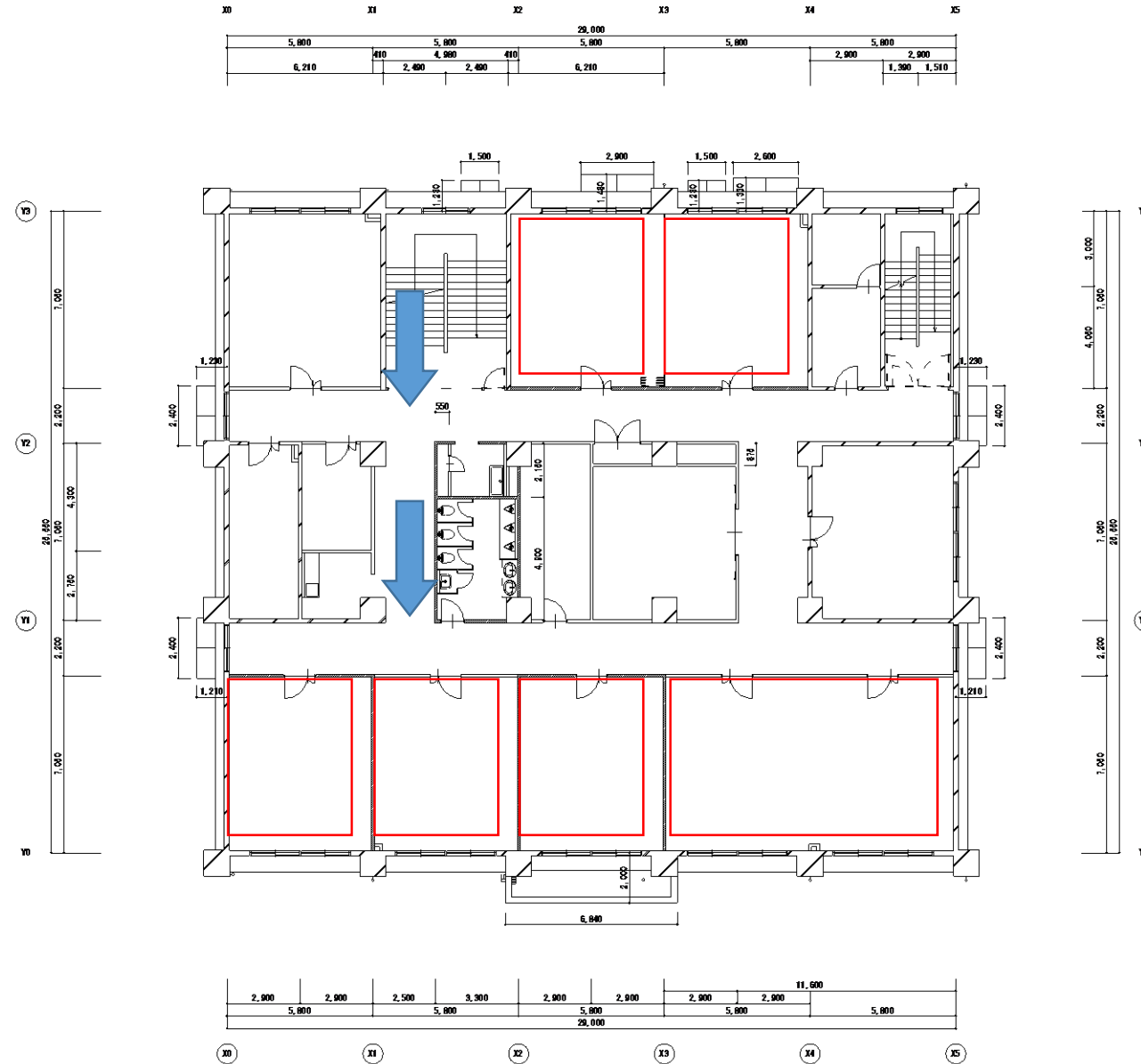
図 3 新隊舎 2 F
