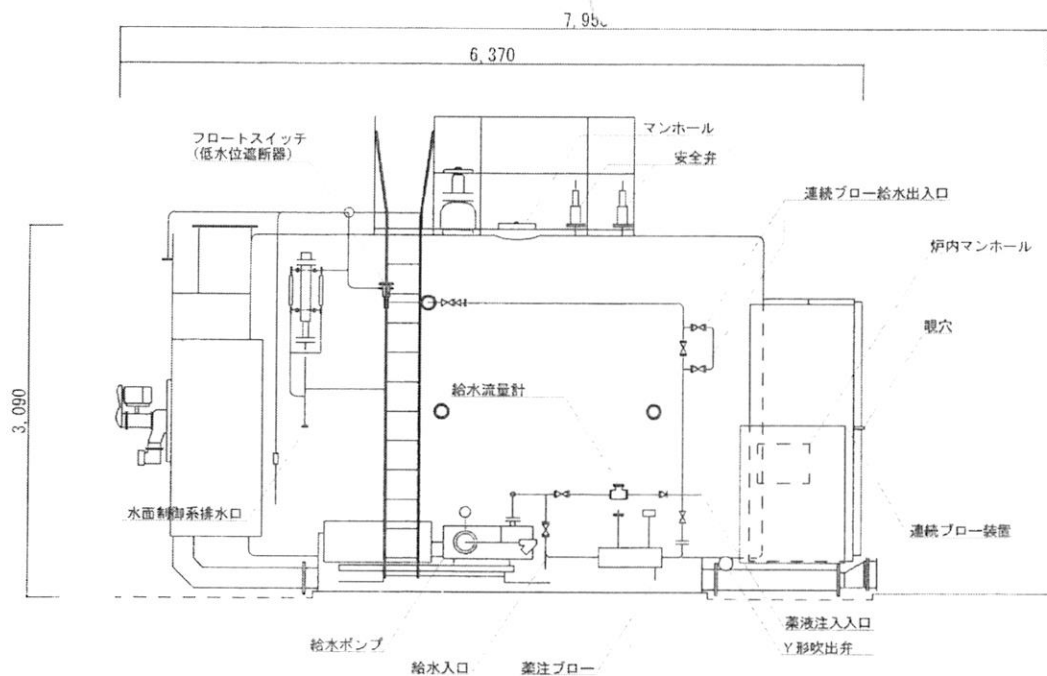
炉筒煙管式ボイラー側面図 A S=1/60
