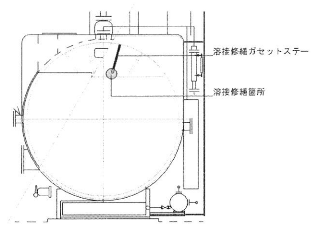
炉筒煙管式ボイラー側面図 B S=1/60
