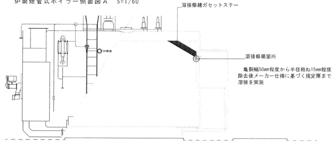
炉筒煙管式ボイラー断面図 A S=1/60
