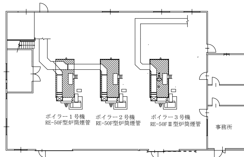
ボイラー室平面図 S=1/250
