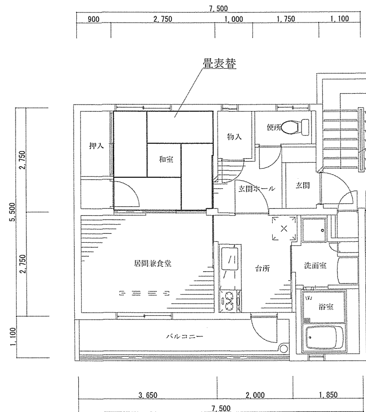
黒鳥宿舎2棟平面図 (偶数部屋) S=1/100
