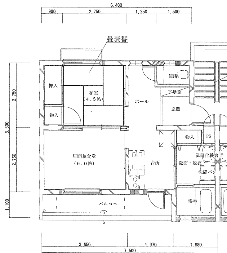
黒鳥宿舎1棟平面図 (偶数部屋) S=1/100
