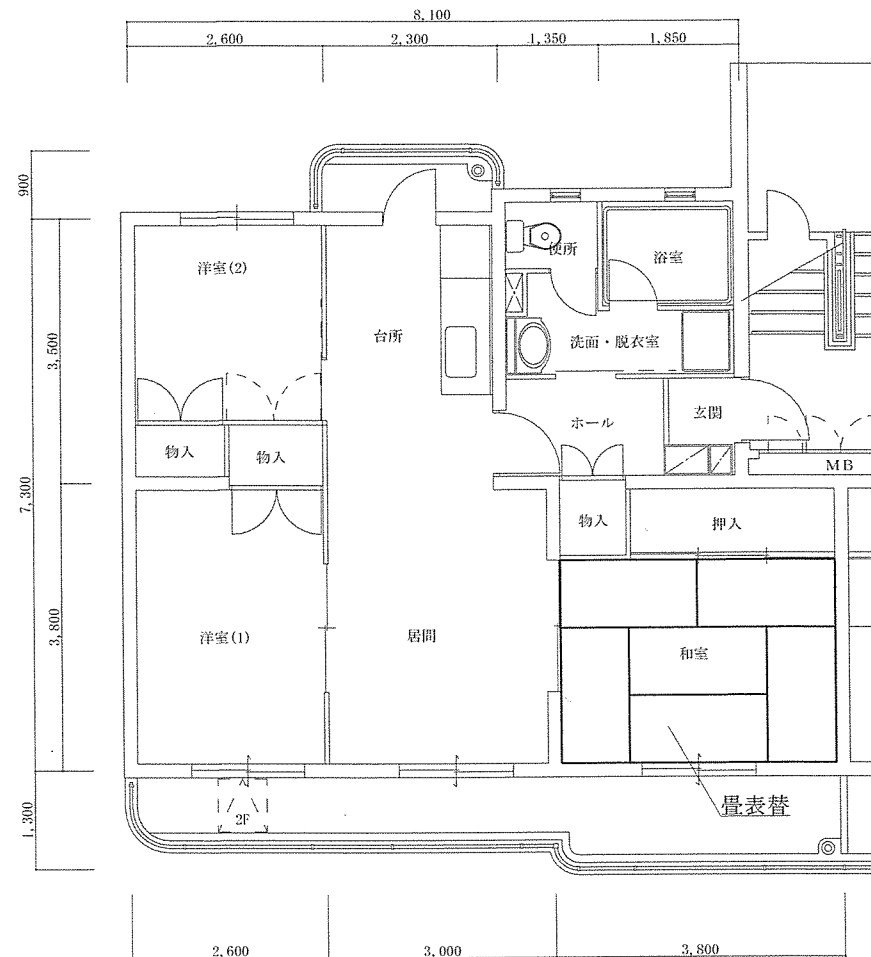
黒鳥宿舎 7 棟 (偶数部屋) S=1/100
