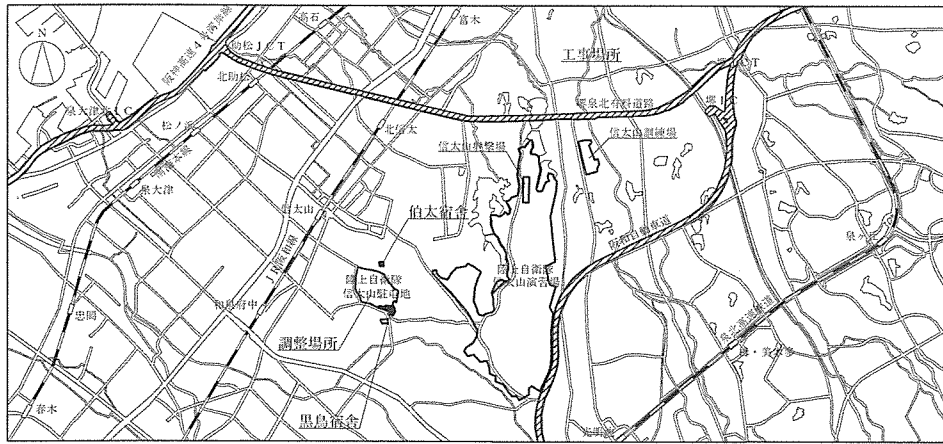
案内図 S-1/100,000
