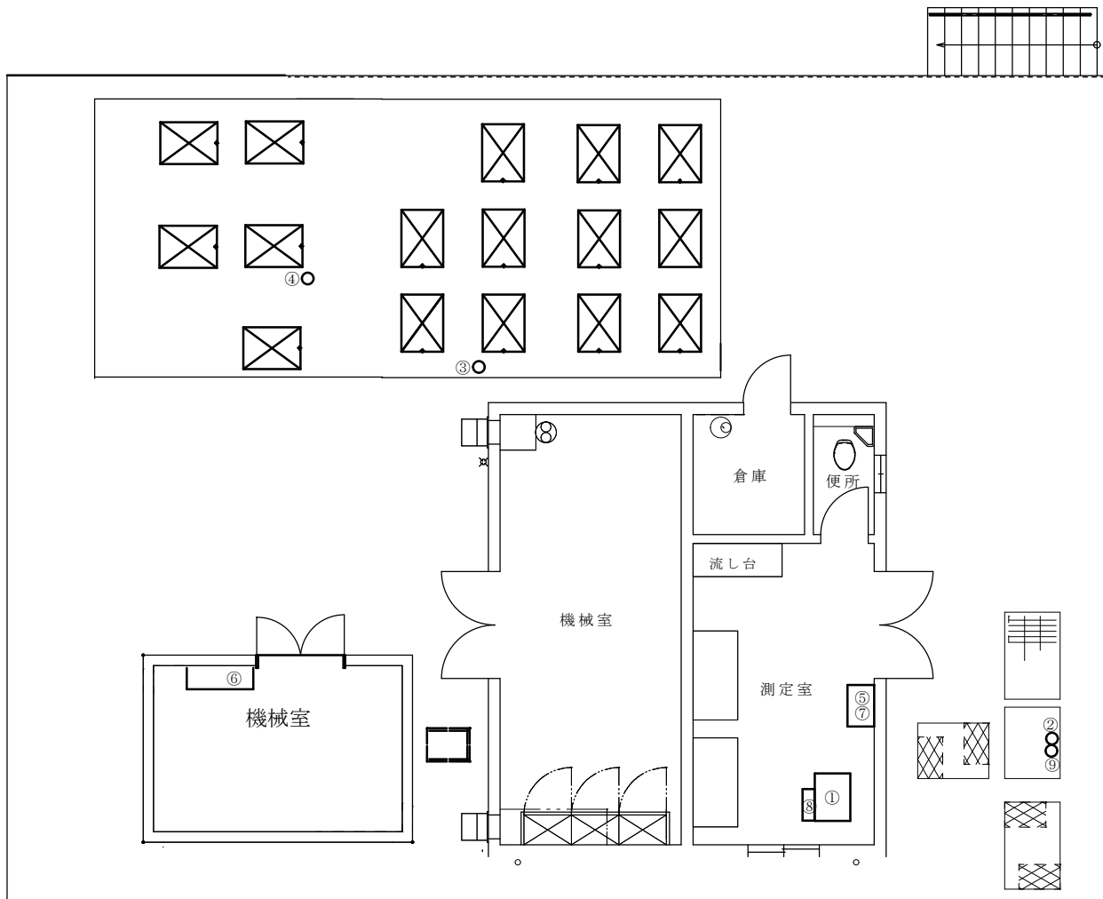
配置図
